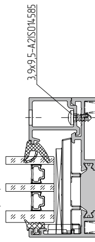
Схема крепления профиля штапика винтами самонарезающими 3,9x9,5-A2IS014585
