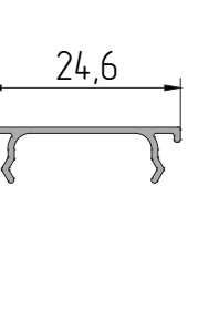
AYPC.T11.0605 Профиль крыши P = 79,3 мм
