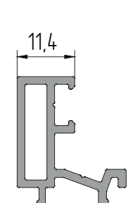
AYPC.W62.0603 Профиль штапика P = 133,2 мм
