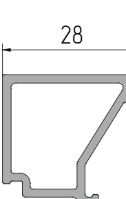
AYPC.C48.2607 Профиль штапика P = 108 мм
