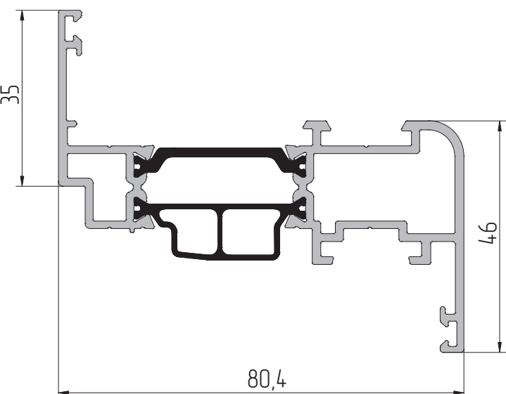
AYPC.W72.3.0303 Профиль импоста P = 487 мм J x = 34,9 см² J y = 26,3 см²
