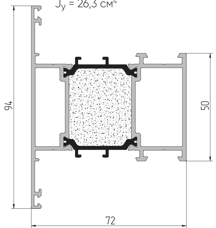
AYPC.W72.3.0303 Профиль импоста P = 487 мм J x = 34,9 см² J y = 26,3 см²
