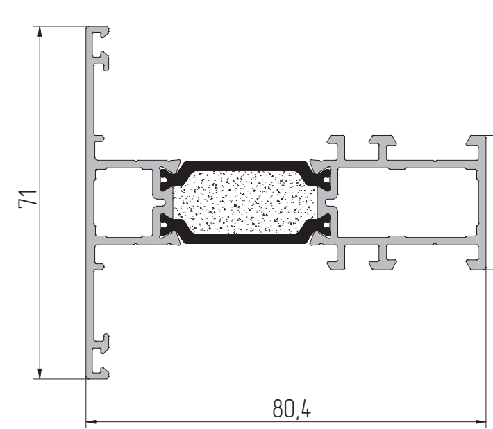
AYPC.W72.3.0840 Профиль соединителя P = 583 мм J x = 74,0 см² J y = 99,24 см²
