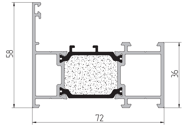
AYPC.W72.3.0202 Профиль створки P = 444 мм J x = 36,5 см² J y = 14,4 см²
