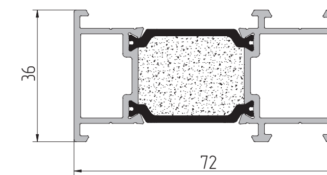
AYPC.W72.3.0122 Профиль уширителя P = 296 мм J x = 21,3 см² J y = 4,9 см²
