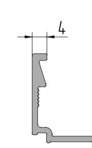
AYPC.C48.0601A Профиль штапика P = 96,1 мм
