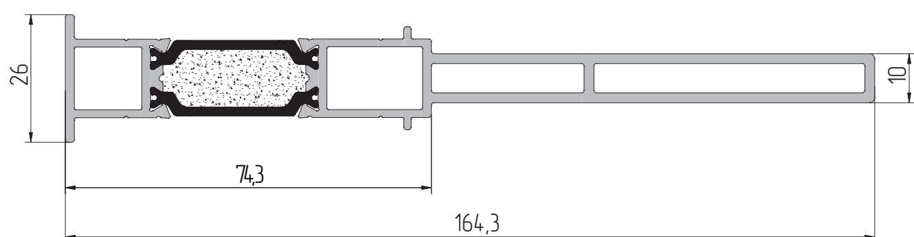
AYPC.W62.0602 Профиль штапика P = 75,1 мм
