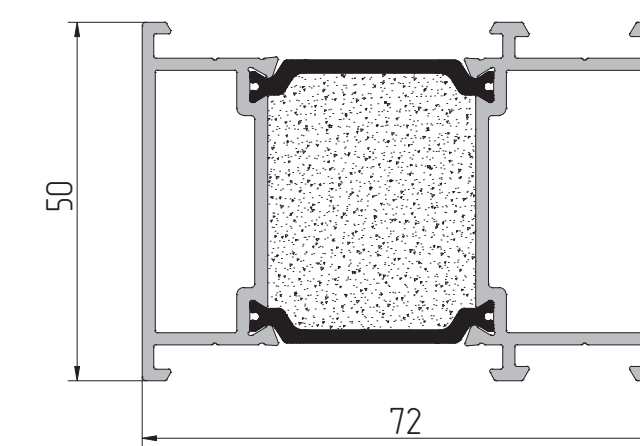
AYPC.W72.3.0123 Профиль уширителя P = 324 мм J x = 27,8 см² J y = 13,2 см²
