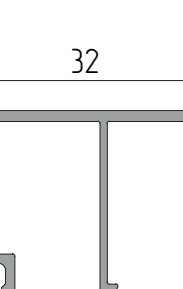
AYPC.C48.0608A Профиль штапика P = 189,1 мм
