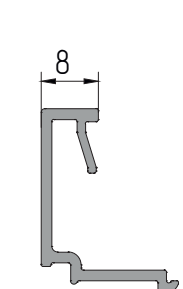
AYPC.C48.0602A Профиль штапика P = 117,7 мм
