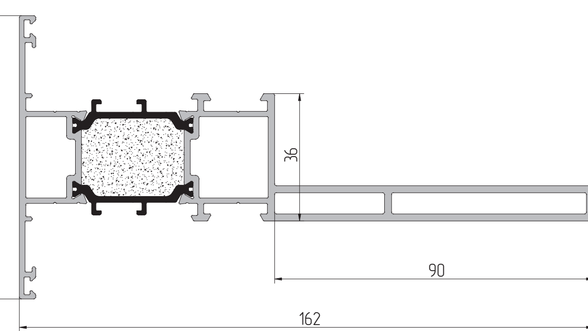
AYPC.W72.3.0304 Профиль импоста P = 638 мм J x = 171,9 см² J y = 17,9 см²
