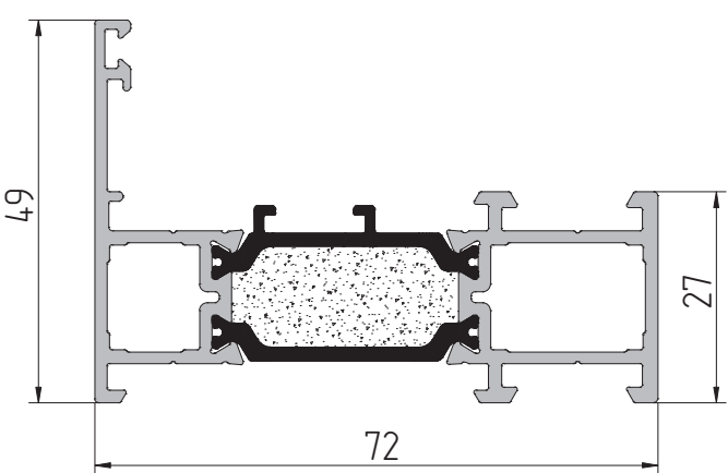
AYPC.W72.3.0201 Профиль створки P = 413 мм J x = 30,6 см² J y = 8,2 см²
