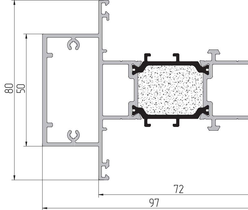
AYPC.W72.3.0841 Профиль соединителя P = 583 мм J x = 70,0 см² J y = 92,86 см²
