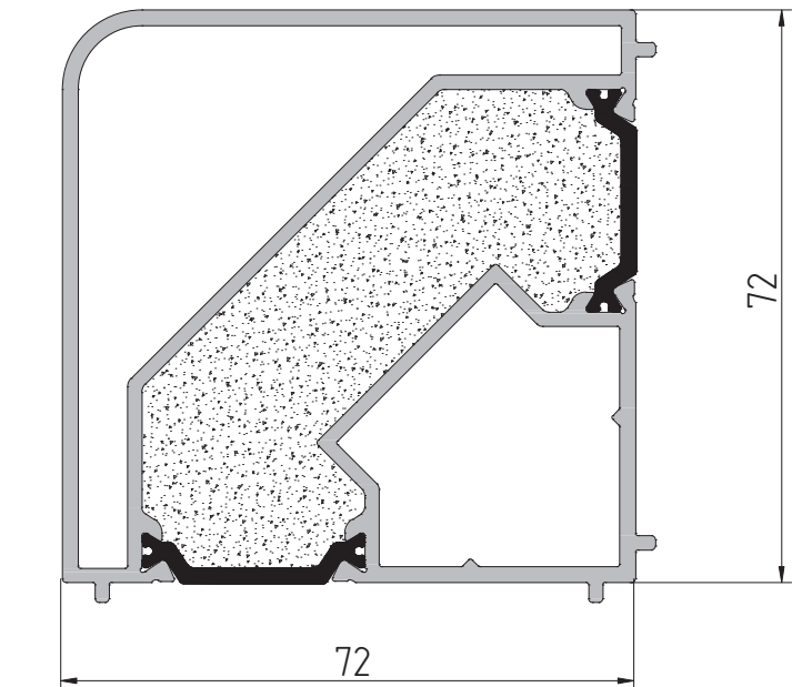
AYPC.BF73.0414 Профиль отлива P = 541,3 мм
