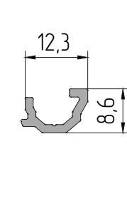
AYPC.W62.0604 Профиль штапика P = 50,8 мм
