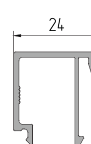
AYPC.C48.0606A Профиль штапика P = 173,1 мм
