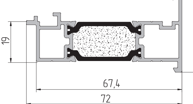
AYPC.C48.0601 Профиль штапика P = 95,3 мм
