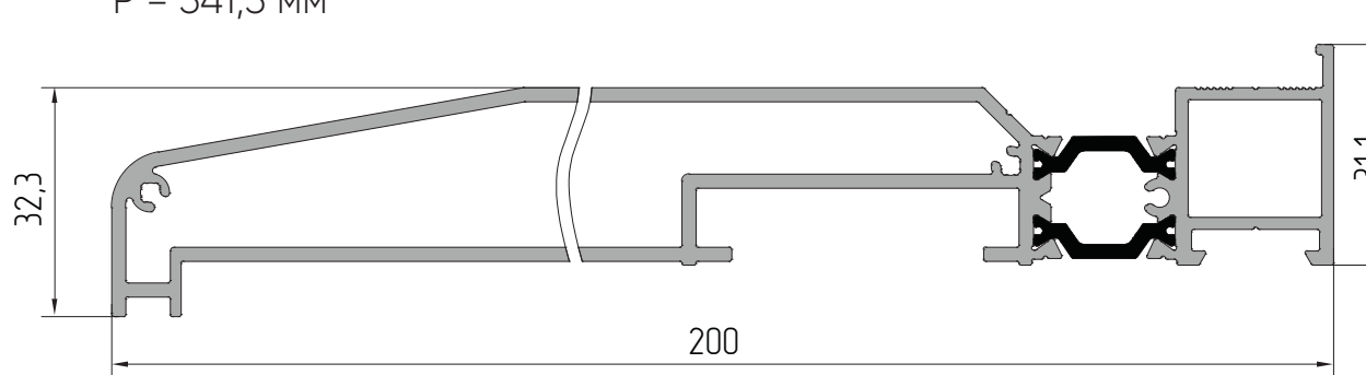
AYPC.W72.0921 Профиль адаптера универсальный
