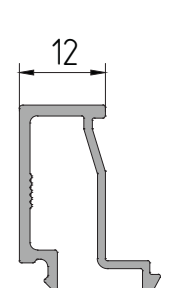
AYPC.C48.0603A Профиль штапика P = 146,1 мм
