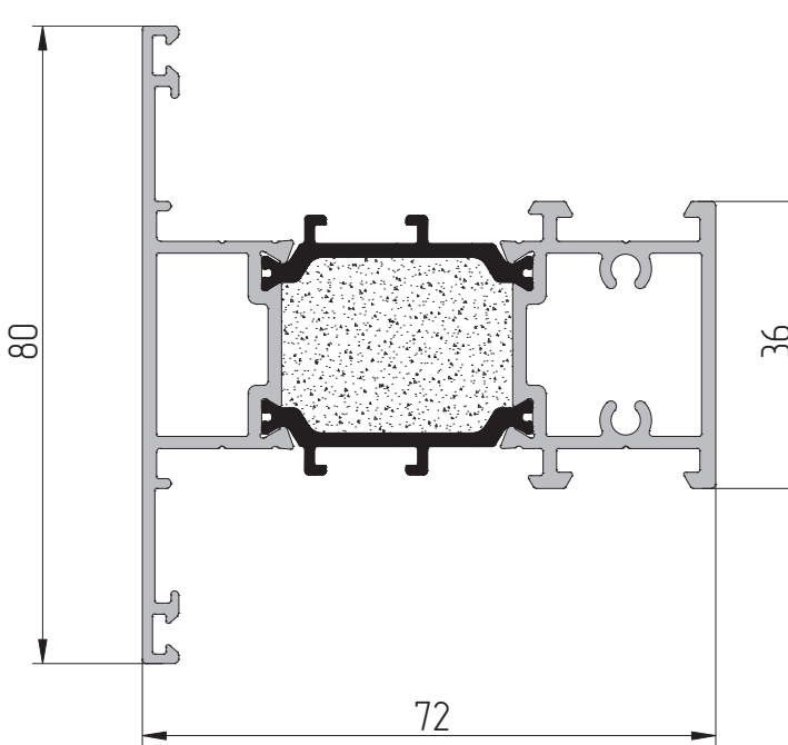
AYPC.W72.3.0315 Профиль импоста P = 509,9 мм J x = 30,22 см² J y = 13,91 см²
