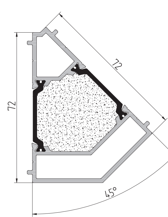
AYPC.W72.3.0849 Профиль соединителя P = 225 мм J x = 20,5 см² J y = 14,81 см²
