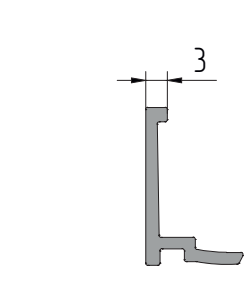
AYPC.W62.0602 Профиль штапика P = 75,1 мм
