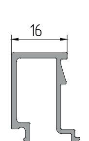
AYPC.C48.0604A Профиль штапика P = 150,7 мм
