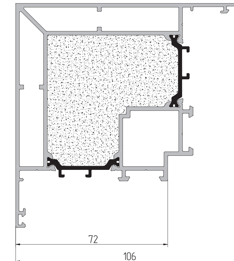
AYPC.C48.0606 Профиль штапика P = 172,2 мм
