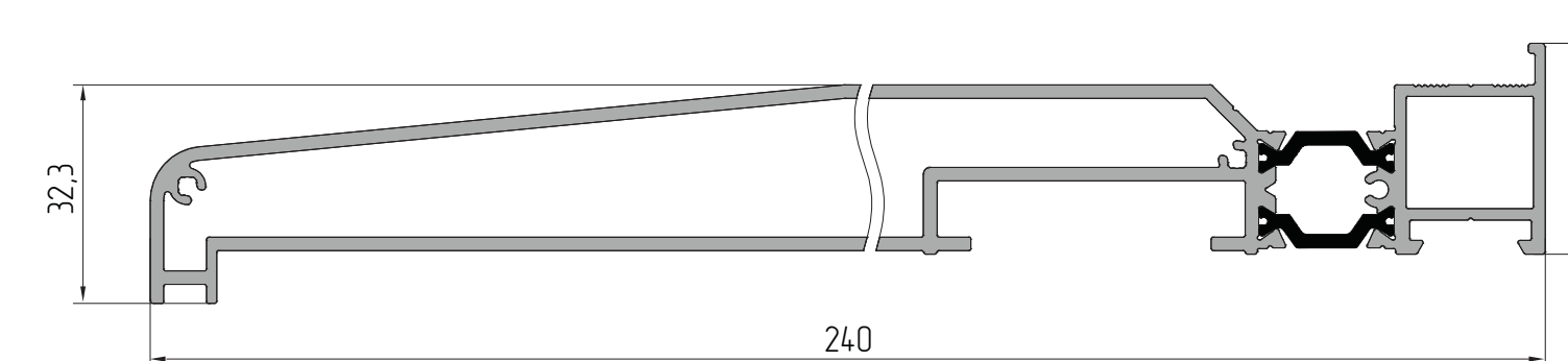
AYPC.C48.0637 Профиль штапика P = 197,3 мм
