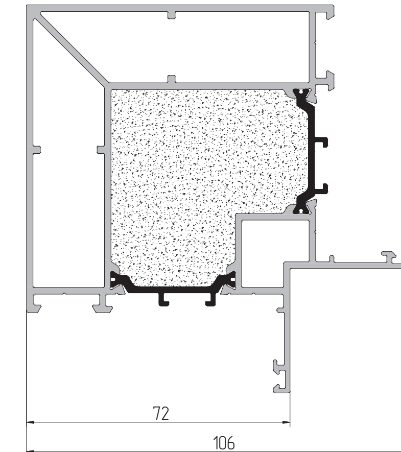
AYPC.C48.0608 Профиль штапика P = 188,2 мм
