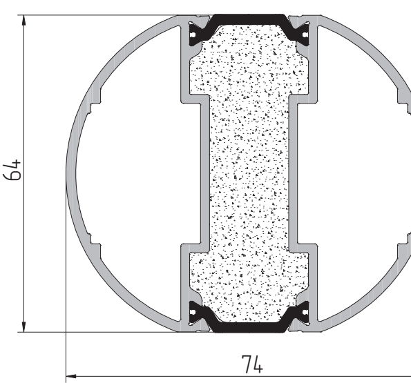
AYPC.W72.3.0805 Профиль соединителя P = 231 мм J x = 24,3 см² J y = 26,6 см²
