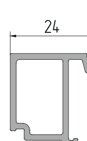
AYPC.C48.2606 Профиль штапика P = 112 мм
