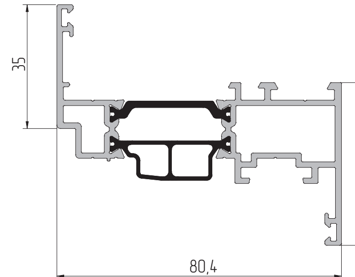
AYPC.W72.3.0315 Профиль импоста P = 509,9 мм J x = 30,22 см² J y = 13,91 см²
