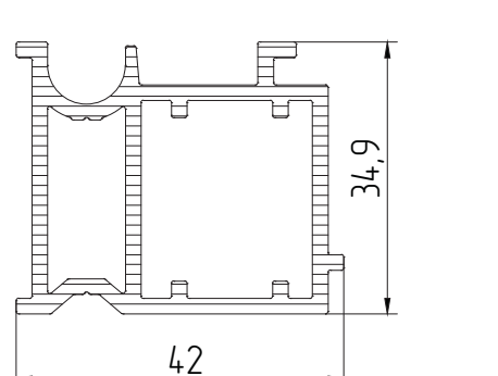
AYPC.F50.0702 Профиль вспомогательный P = 76,7 мм
