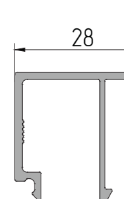
AYPC.C48.0607A Профиль штапика P = 181,1 мм
