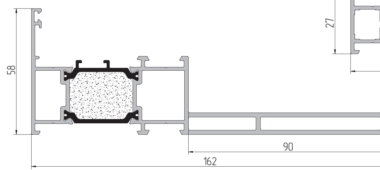
AYPC.W72.3.0222 Профиль створки P = 457,2 мм J x = 37,0 см² J y = 14,48 см²
