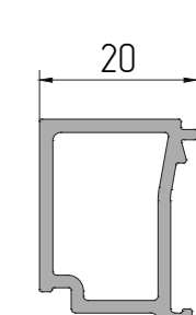
AYPC.C48.2605 Профиль штапика P = 97 мм
