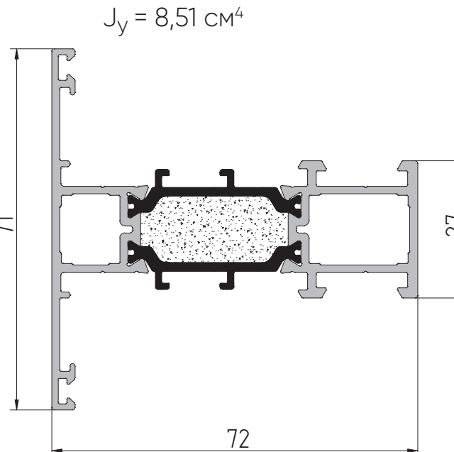
AYPC.W72.3.0301 Профиль импоста P = 421 мм J x = 24,3 см² J y = 8,51 см²
