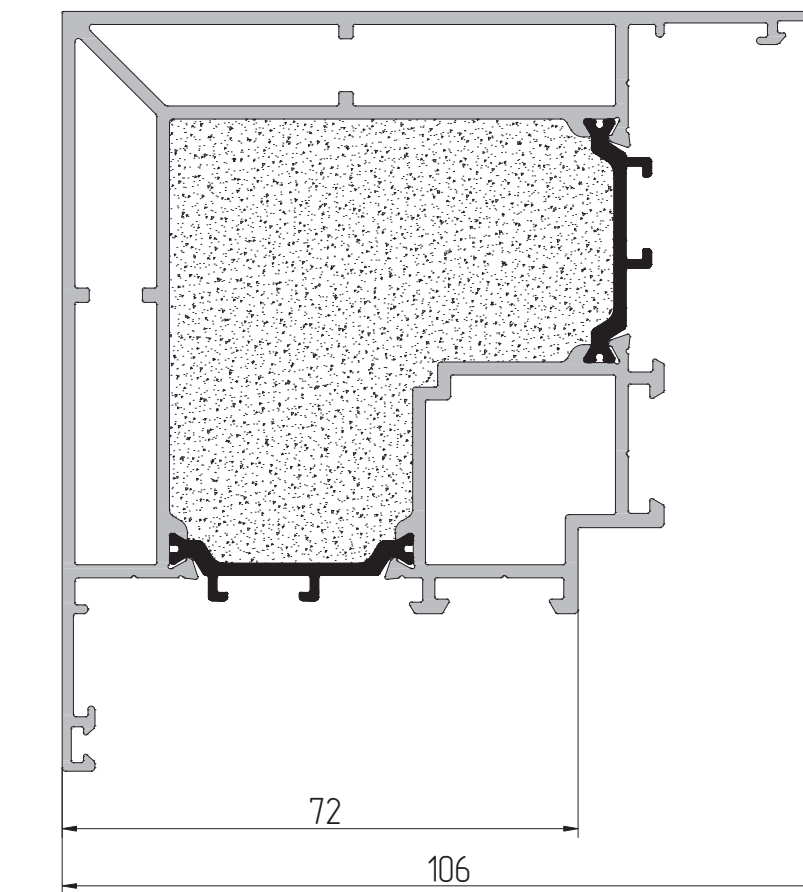
AYPC.C48.0606 Профиль штапика P = 172,2 мм
