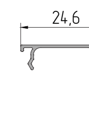
AYPC.T11.0605 Профиль крыши P = 79,3 мм
