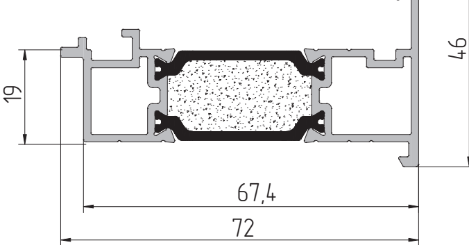
AYPC.C48.0601 Профиль штапика P = 95,3 мм
