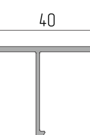
AYPC.C48.0636A Профиль штапика P = 205,3 мм
