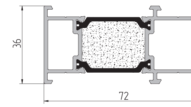
AYPC.W72.3.0122 Профиль уширителя P = 296 мм J x = 21,3 см² J y = 4,9 см²
