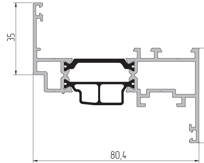
AYPC.W72.3.0315 Профиль импоста P = 509,9 мм J x = 30,22 см² J y = 13,91 см²
