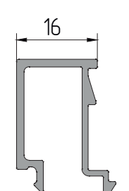
AYPC.C48.0604A Профиль штапика P = 150,7 мм
