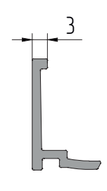
AYPC.W62.0602 Профиль штапика P = 75,1 мм
