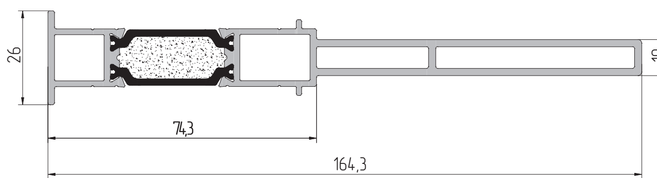
AYPC.W62.0602 Профиль штапика P = 75,1 мм
