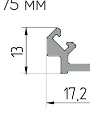
AYPC.W62.0607 Профиль тяги P = 39,2 мм
