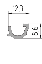
AYPC.W62.0604 Профиль штапика P = 50,8 мм
