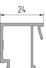
AYPC.C48.0606A Профиль штапика P = 173,1 мм
