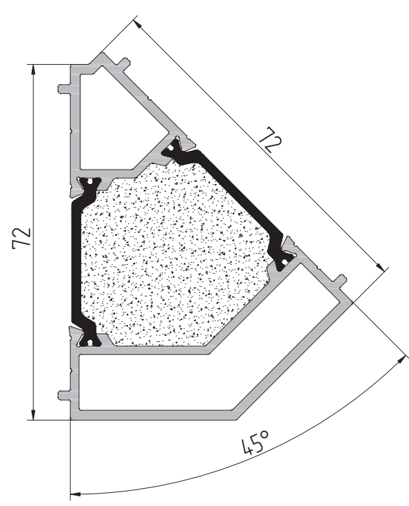
AYPC.C48.0604 Профиль штапика P = 151 мм
