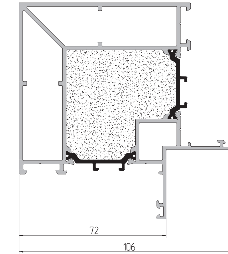
AYPC.C48.0608 Профиль штапика P = 188,2 мм
