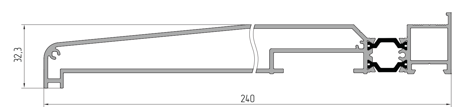
AYPC.C48.0637 Профиль штапика P = 197,3 мм
