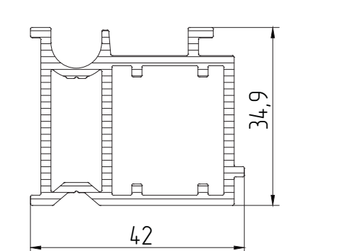
AYPC.F50.0702 Профиль вспомогательный P = 76,7 мм
