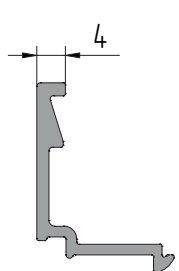
AYPC.C48.0601A Профиль штапика P = 96,1 мм
