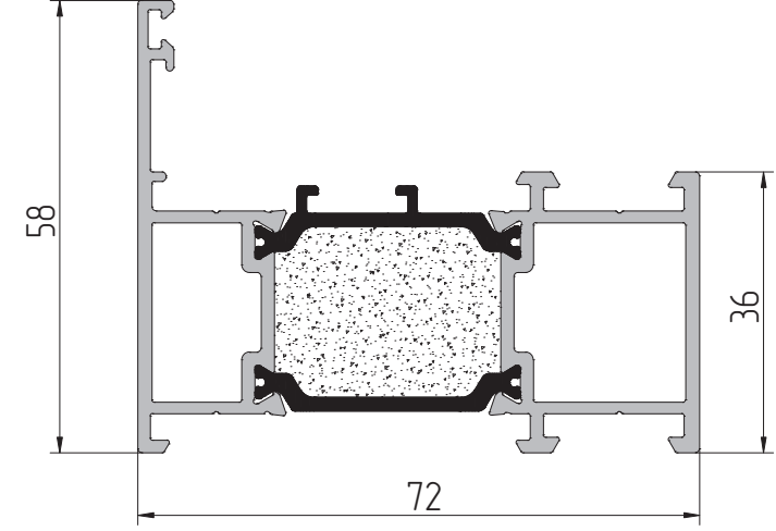
AYPC.W72.3.0202 Профиль створки P = 444 мм J x = 36,5 см² J y = 14,4 см²
