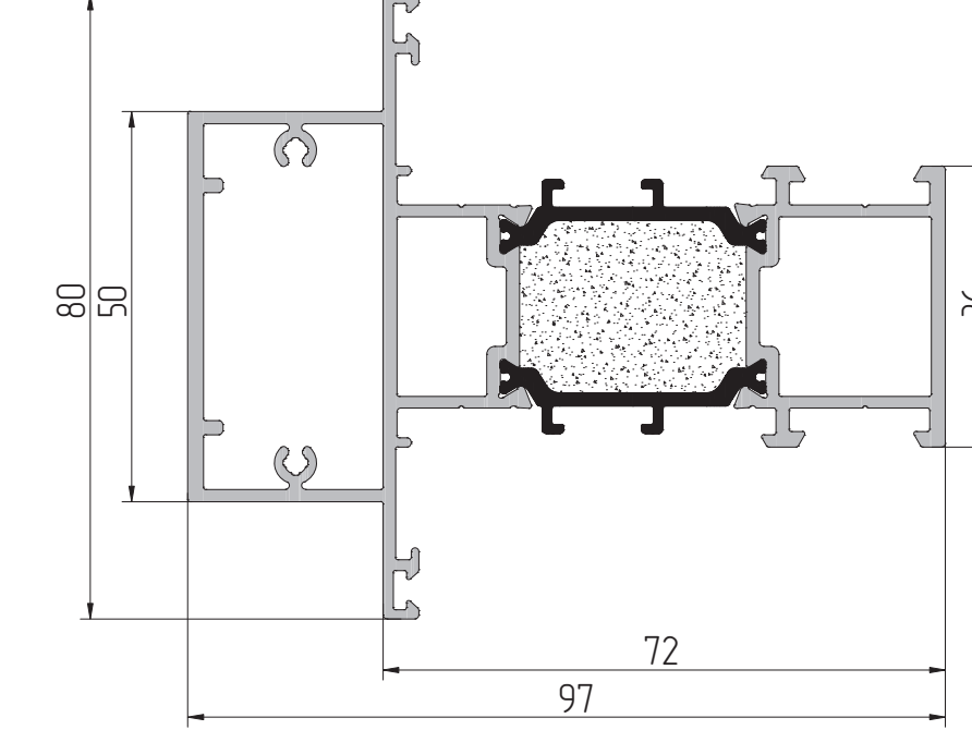
AYPC.W72.3.0841 Профиль соединителя P = 583 мм J x = 70,0 см² J y = 92,86 см²
