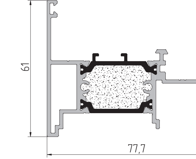
AYPC.W72.3.0504 Профиль штапика P = 411 мм J x = 22,41 см² J y = 7,54 см²
