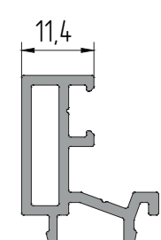
AYPC.W62.0603 Профиль штапика P = 133,2 мм
