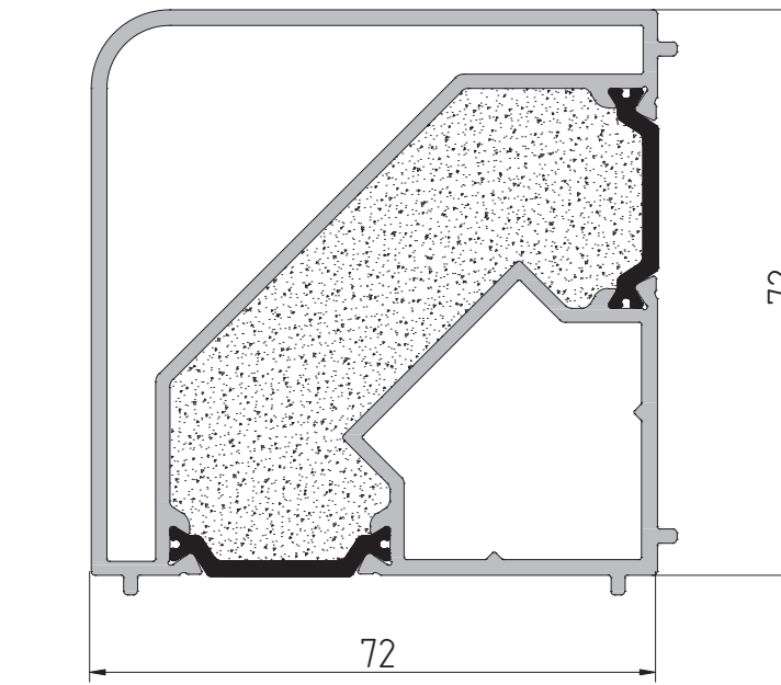
AYPC.BF73.0414 Профиль отлива P = 541,3 мм
