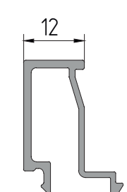
AYPC.C48.0603A Профиль штапика P = 146,1 мм
