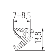
FRK231 Уплотнитель резиновый
