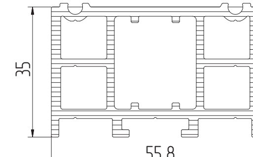
AYPC.W72.9907 Профиль адаптера универсальный
