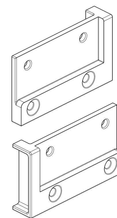
AYPC.W72.9904K Комплект заглушек порога
