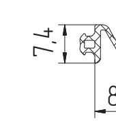
FRK211 Уплотнитель резиновый
