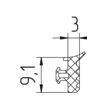
FRK29-01 Уплотнитель резиновый
