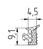
FRK197 Уплотнитель резиновый
