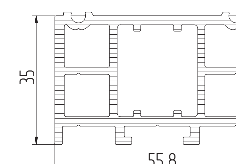
AYPC.W72.9907 Профиль адаптера универсальный
