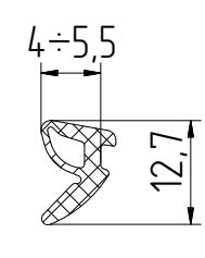
FRK191 Уплотнитель резиновый
