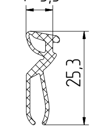
FRK193 Уплотнитель резиновый
