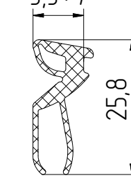
FRK194 Уплотнитель резиновый
