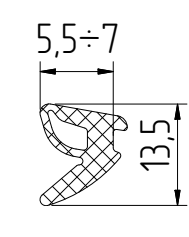
FRK192 Уплотнитель резиновый
