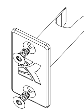
AYPC.W62.9912K Комплект элемента регулирующего
