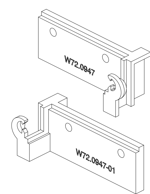
AYPC.W72.0947K Комплект заглушек порога
