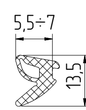
FRK192 Уплотнитель резиновый
