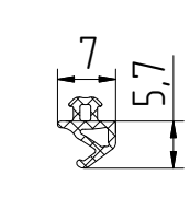
FRK198 Уплотнитель резиновый
