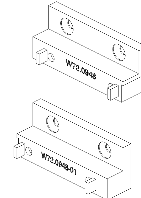
AYPC.W72.0948K Комплект заглушек порога
