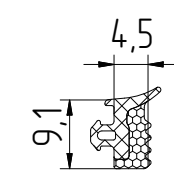
FRK197 Уплотнитель резиновый
