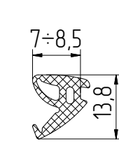
FRK231 Уплотнитель резиновый
