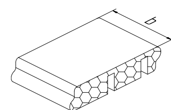
AYPC.W62.0916 b = 22 мм AYPC.W62.0916-01 b = 32 мм AYPC.W62.0916-02 b = 45 мм Подкладка
