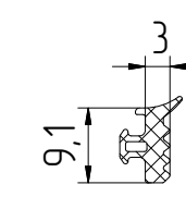
FRK29-01 Уплотнитель резиновый
