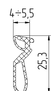
FRK193 Уплотнитель резиновый
