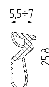
FRK194 Уплотнитель резиновый
