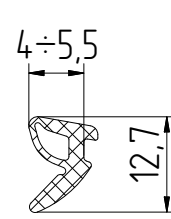
FRK191 Уплотнитель резиновый
