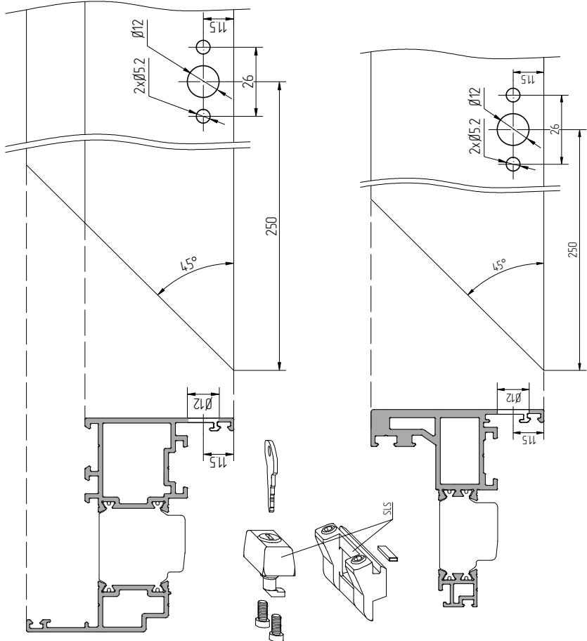
Обработка профиля створки под установку SLS
