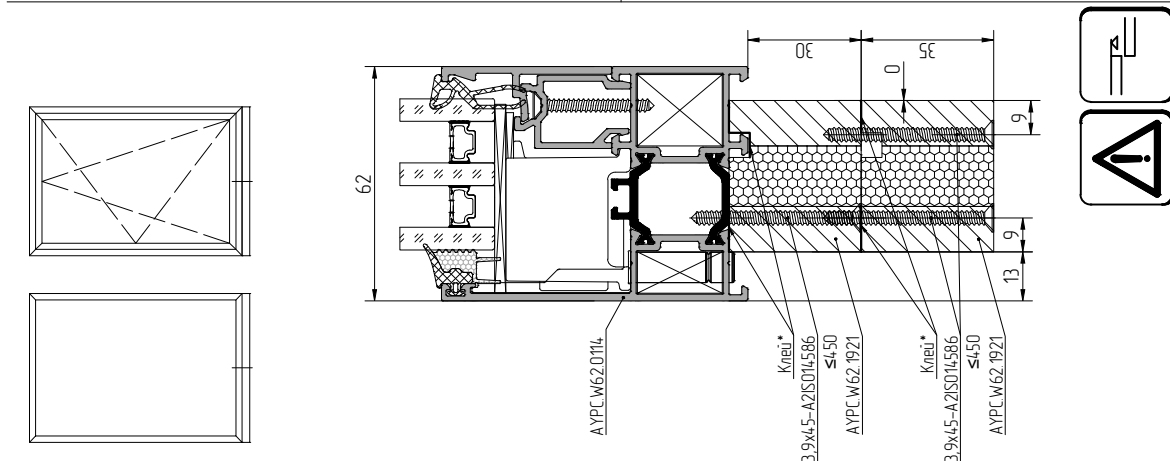
Схема установки и фиксации подставочного профиля АУРС W62.1921 по низу конструкции
