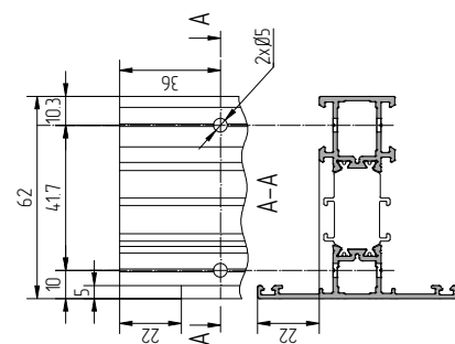
Схема обработки АУРС.W62.0301, АУРС.W62.0302, АУРС.W62.0303, АУРС.W62.0315
