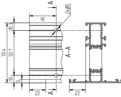
Схема обработки АУРС.W62.0321
