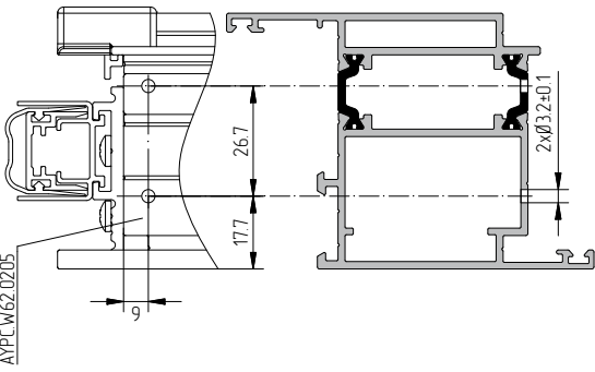
Схема обработки профиля сборки АУРС W62.0205 под установку манжеты ЕРДМ АУРС W62.0926
