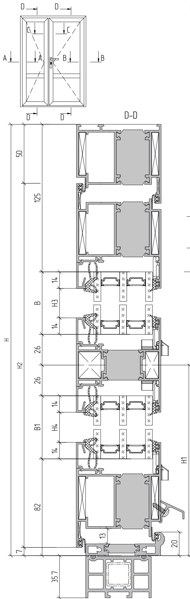
Пример расчета двуствольной двери открыванием внутрь
