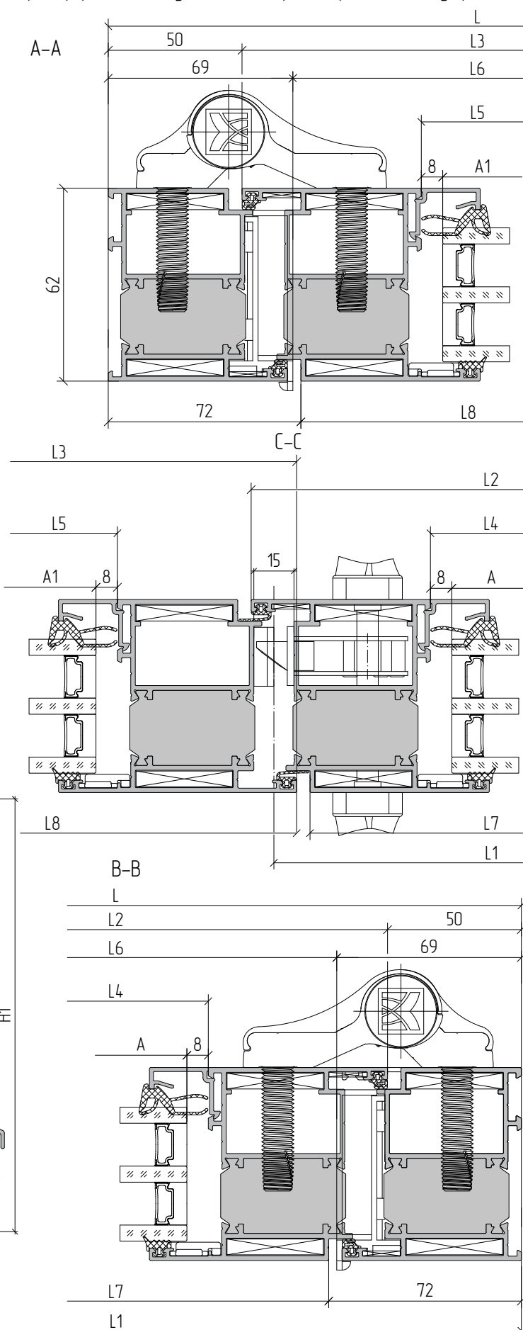
Пример расчета двуствольной двери открыванием внутрь
