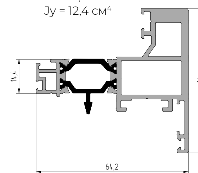
AYPC.W62.0224 Профиль створки P = 373,7 мм Jx = 15,2 см 2 Jy = 12,4 см 2
