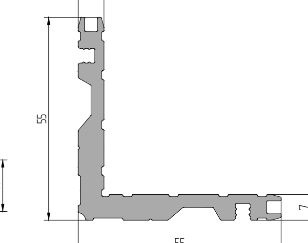
AYPC.W62.0702 Профиль угловой обжимной P = 265,7 мм
