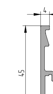
AYPC.W72.0614 Профиль штапика P = 138,4 мм
