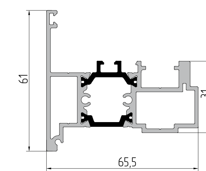
AYPC.W62.0507 Профиль штапика P = 359,9 мм Jx = 20,4 см 2 Jy = 8,6 см 2
