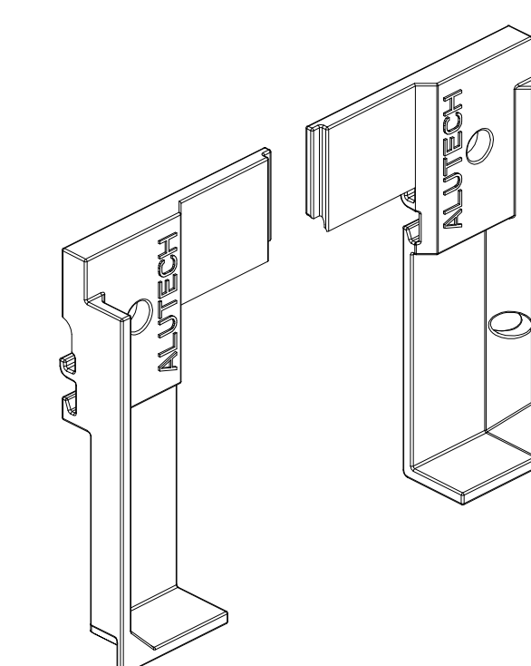
AYPC.W62.0943K Комплект заглушек
