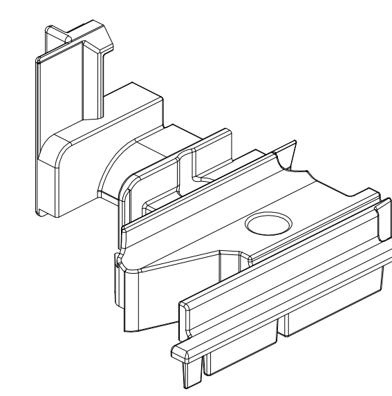
AYPC.W62.0310 Профиль импоста P = 537,2 мм Jx = 23,5 см 2 Jy = 42,1 см 2
