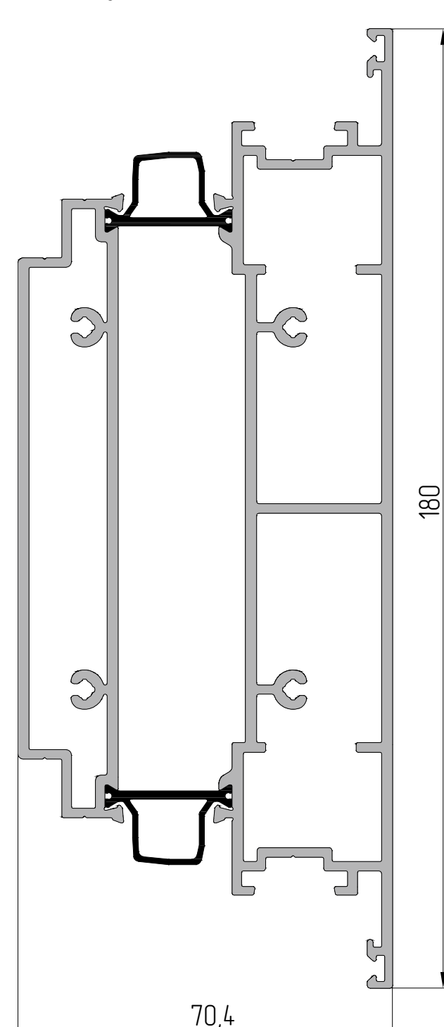
AYPC.W62.0226 Профиль створки P = 682,2 мм Jx = 69,27 см 2 Jy = 312,32 см 2
