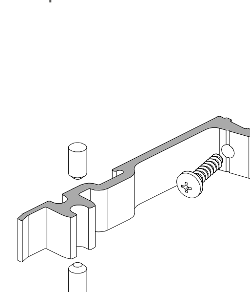
AYPC.W62.0967K Комплект закладной крепления импоста
