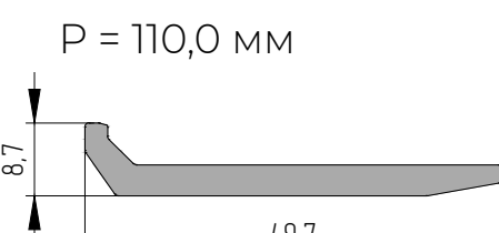
AYPC.F50.0805 Профиль опорный под стеклопакет P = 110,0 мм
