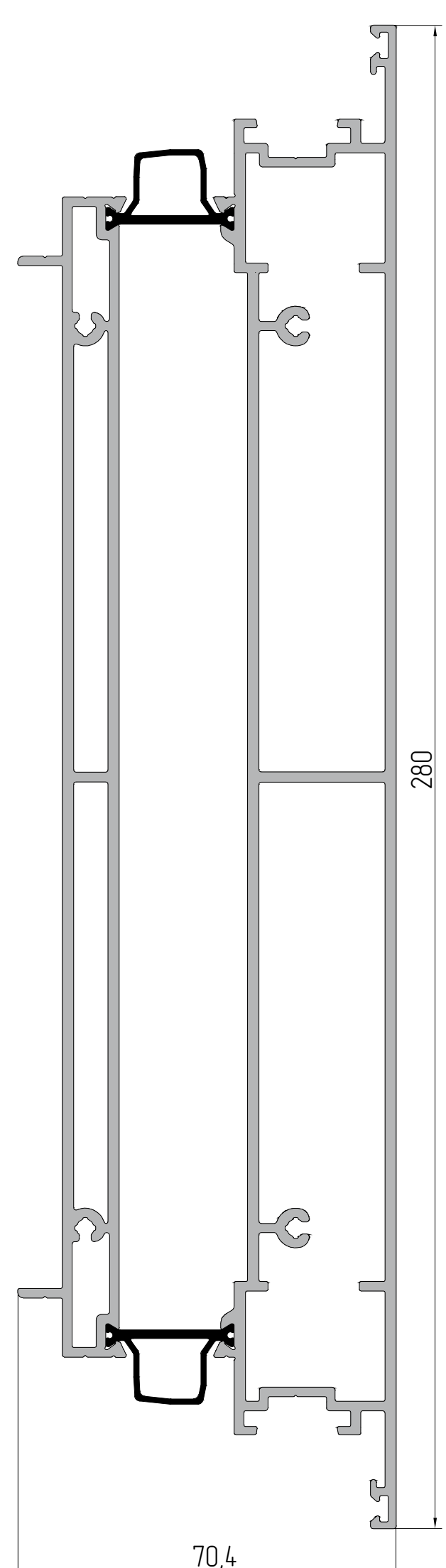
AYPC.W62.0217 Профиль створки P = 896,9 мм Jx = 95,22 см 2 Jy = 1328,14 см 2
