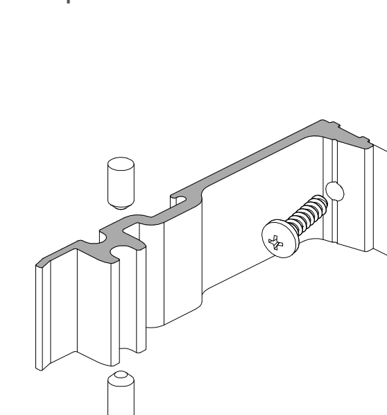
AYPC.W62.0967K-01 Комплект закладной крепления импоста
