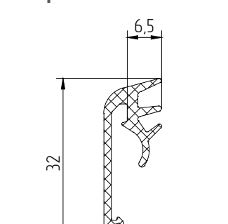
FRK97 Уплотнитель резиновый
