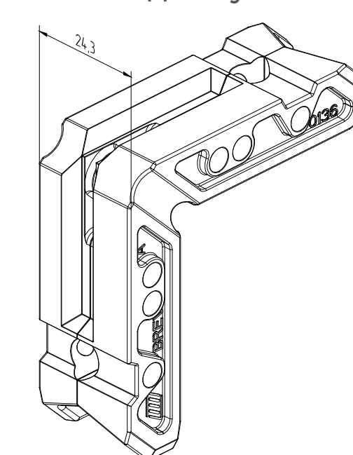
0136/200 Закладная угловая
