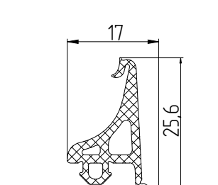
FRK173 Уплотнитель резиновый
