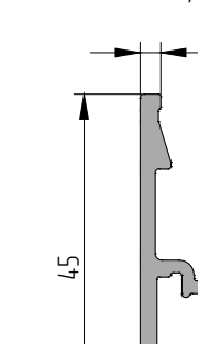
AYPC.W72.0613 Профиль штапика P = 135,4 мм
