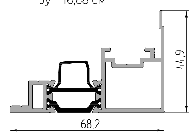
AYPC.W62.0218 Профиль створки P = 896,9 мм Jx = 3,06 см 2 Jy = 16,68 см 2
