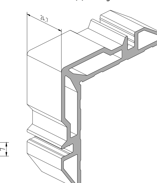
AYPC.W62.0983 Закладная угловая
