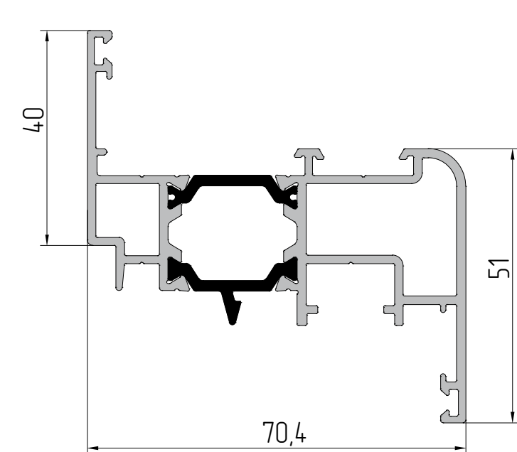
AYPC.W62.0248 Профиль створки P = 435,3 мм Jx = 27,3 см 2 Jy = 10,3 см 2
