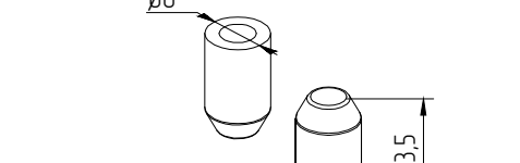
0136/200 0097/400 Штифт для угловой закладной
