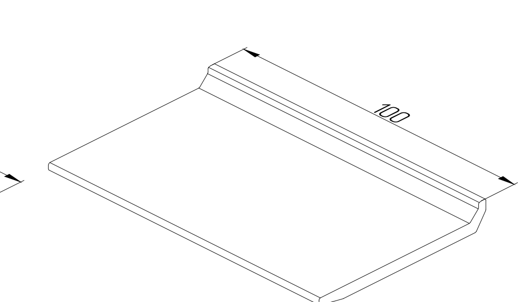
AYPC.F50.0952 Подкладка опорная
