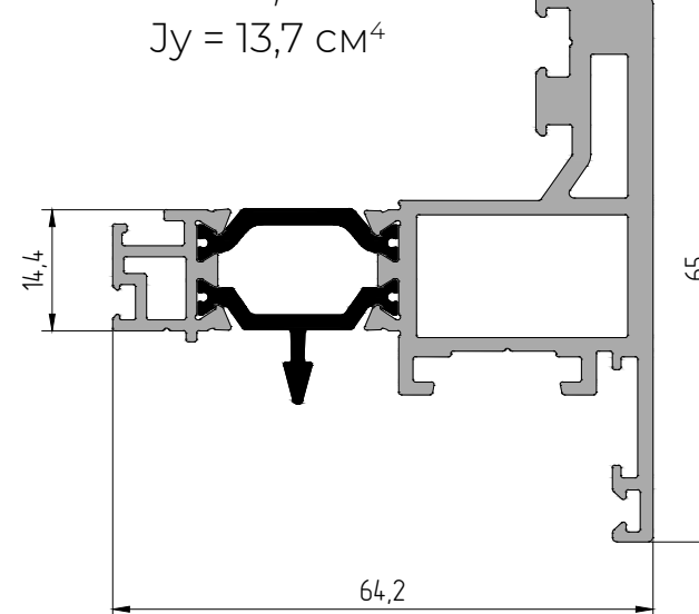
AYPC.W62.0208 Профиль створки P = 379,5 мм Jx = 15,8 см 2 Jy = 13,7 см 2
