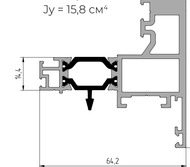
AYPC.W62.0225 Профиль створки P = 381,7 мм Jx = 15,5 см 2 Jy = 15,8 см 2
