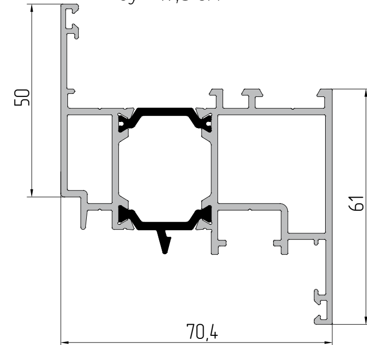
AYPC.W62.0252 Профиль створки P = 466,2 мм Jx = 28,7 см 2 Jy = 17,8 см 2
