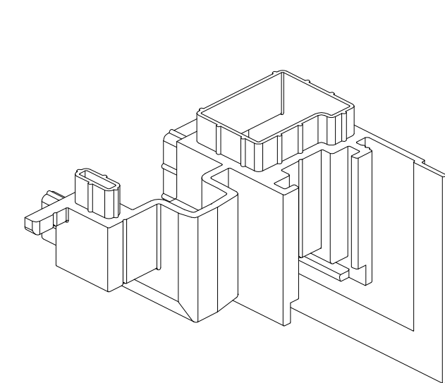
AYPC.W62.0919 Уголок
