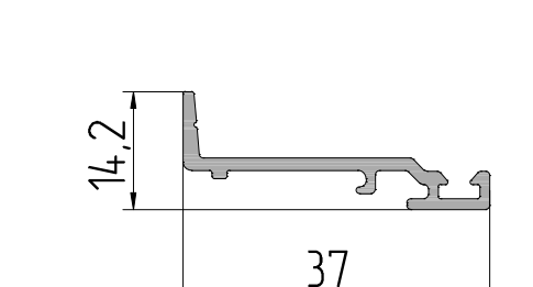
AYPC.W62.0820 Профиль доборный P = 121,7 мм
