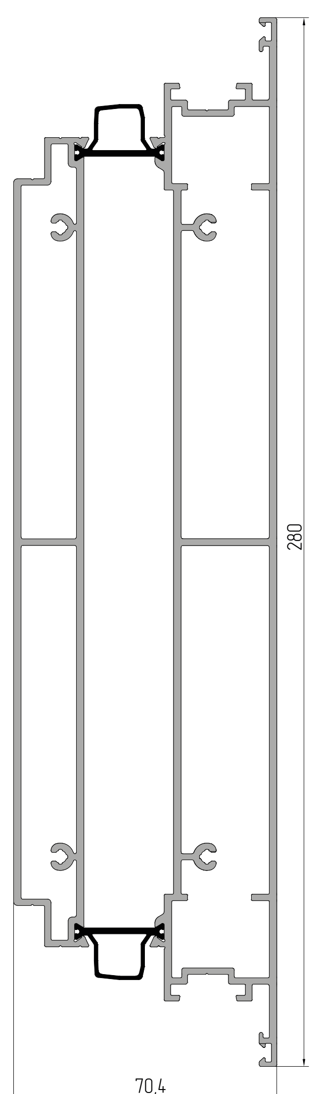
AYPC.W62.0216 Профиль створки P = 880,8 мм Jx = 112,78 см 2 Jy = 1348,03 см 2
