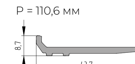
AYPC.F50.0804 Профиль опорный под стеклопакет P = 110,6 мм
