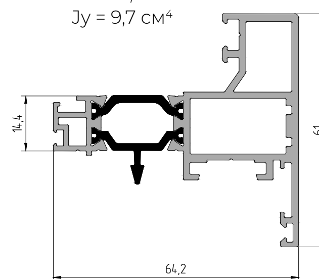
AYPC.W62.0207 Профиль створки P = 372,8 мм Jx = 14,1 см 2 Jy = 9,7 см 2
