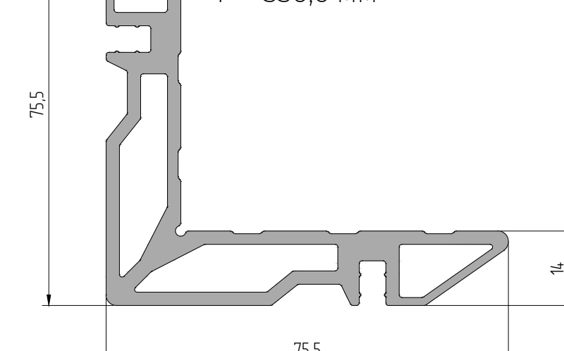
AYPC.100.1504 Профиль алюминиевый экструдированный P = 330,0 мм
