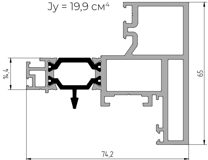
AYPC.W62.0227 Профиль створки P = 400,0 мм Jx = 23,1 см 2 Jy = 19,9 см 2
