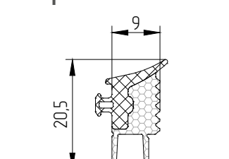
FRK180 Уплотнитель резиновый
