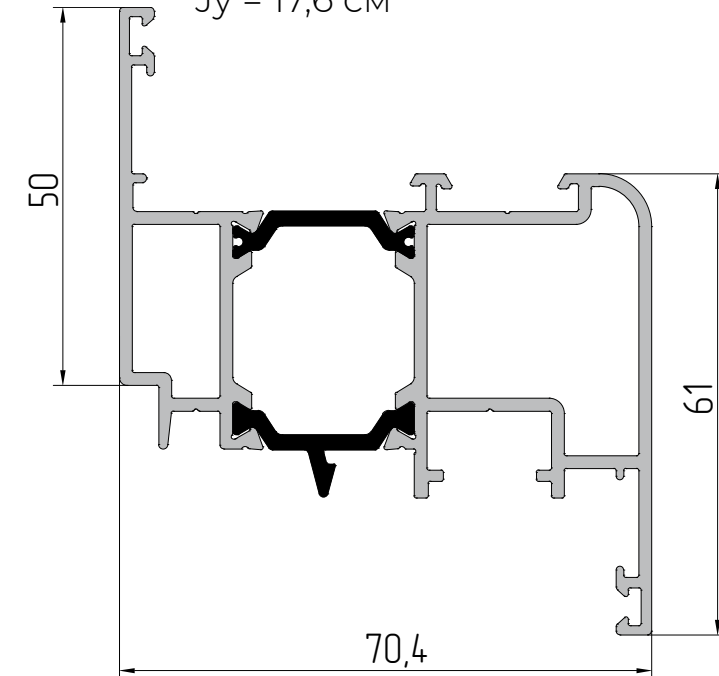
AYPC.W62.0249 Профиль створки P = 455,2 мм Jx = 28,1 см 2 Jy = 17,6 см 2
