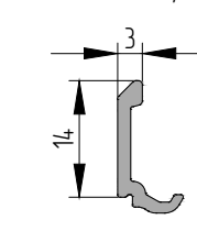
AYPC.W72.0601 Профиль штапика P = 46,7 мм
