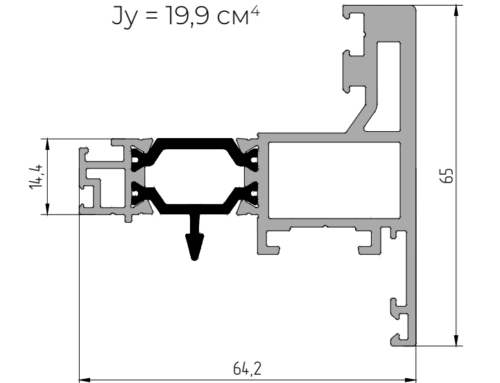
AYPC.W62.0228 Профиль створки P = 450,0 мм Jx = 22,6 см 2 Jy = 19,9 см 2
