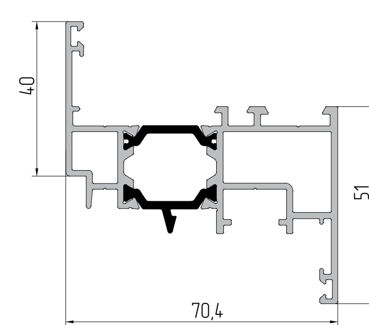
AYPC.W62.0251 Профиль створки P = 446,4 мм Jx = 24 см 2 Jy = 10,4 см 2
