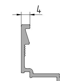
AYPC.C48.0601A Профиль штапика P = 96,1 мм
