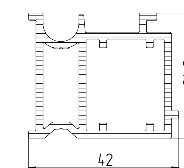
AYPC.C48.0637 Профиль штапика P = 197,3 мм
