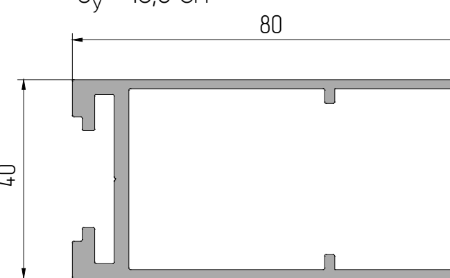
AYPC.C48.0608 Профиль штапика P = 189 мм
