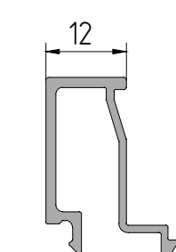
AYPC.C48.0603A Профиль штапика P = 146,1 мм
