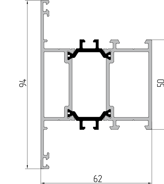
AYPC.W62.0812 Профиль соединителя P = 383 мм J x = 110,1 см² J y = 1,8 см²
