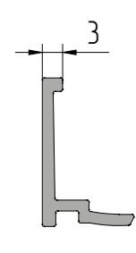
AYPC.W62.0602 Профиль штапика P = 75 мм
