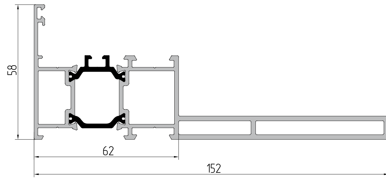
AYPC.W62.0301 Профиль импоста P = 430 мм J x = 17,0 см² J y = 8,5 см²
