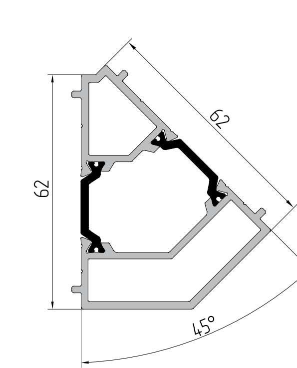
AYPC.W62.0849 Профиль соединителя P = 230 мм J x = 13,2 см² J y = 10,3 см²
