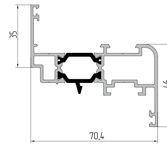
AYPC.W62.0315 Профиль импоста P = 449 мм J x = 20,7 см² J y = 13,9 см²
