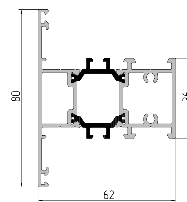
AYPC.W62.0840 Профиль соединителя P = 549 мм J x = 53,0 см² J y = 53,0 см²
