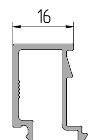
AYPC.C48.0604A Профиль штапика P = 150,7 мм
