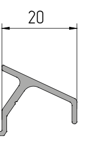
AYPC.C48.2605 Профиль штапика P = 96,5 мм
