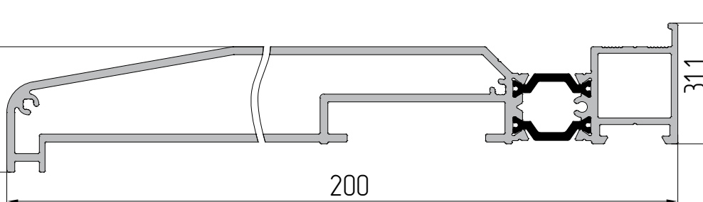
AYPC.C48.0603 Профиль штапика P = 146 мм
