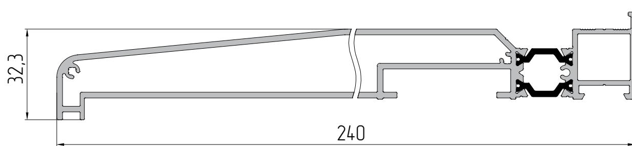
AYPC.C48.0605 Профиль штапика P = 151 мм
