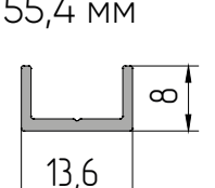
AYPC.C48.0614 Профиль выравнивающий P = 55,4 мм
