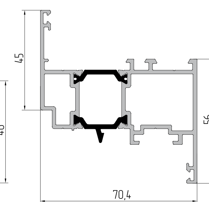
AYPC.W62.0343 Профиль импоста P = 547 мм J x = 84,7 см² J y = 28,7 см²
