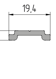
AYPC.C48.0612 Профиль тяги P = 49,3 мм
