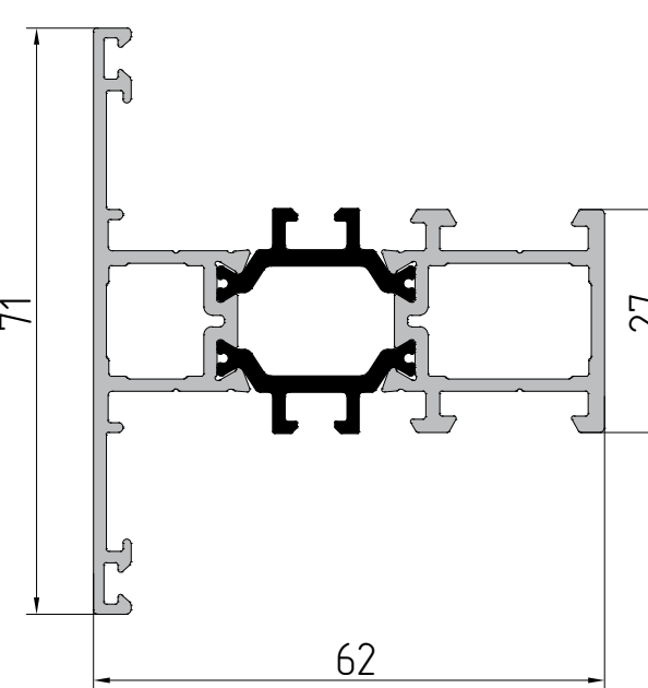
AYPC.W62.0806 Профиль соединителя P = 261 мм J x = 25,1 см² J y = 25,1 см²
