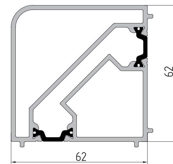
AYPC.W62.0806 Профиль соединителя P = 261 мм J x = 25,1 см² J y = 25,1 см²
