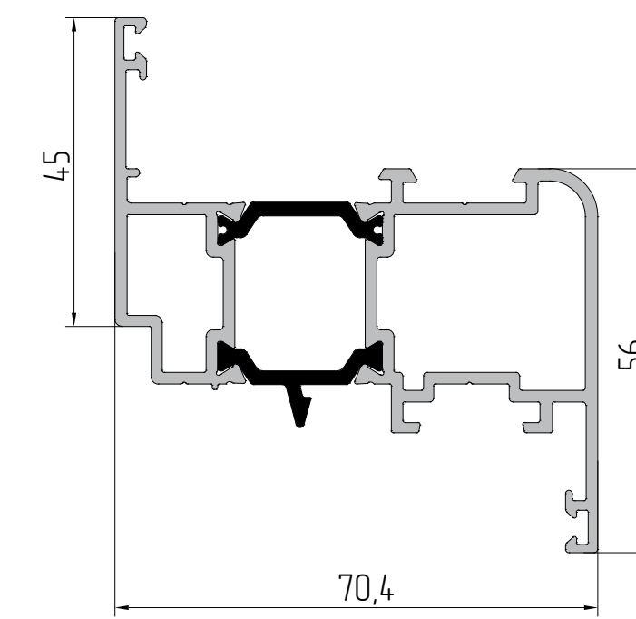
AYPC.W62.0321 Профиль импоста P = 426 мм J x = 22,8 см² J y = 8,9 см²
