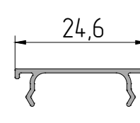
AYPC.T11.0605 Профиль крышки P = 79,3 мм
