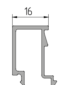
AYPC.C48.0604A Профиль штапика P = 150,7 мм
