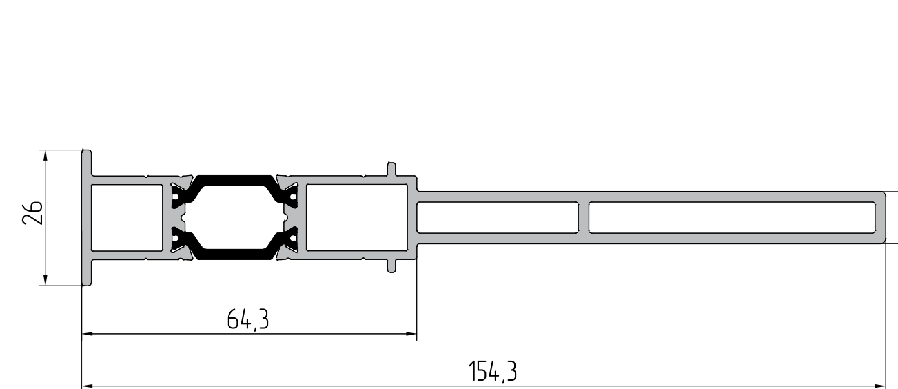
AYPC.W62.0812 Профиль соединителя P = 383 мм J x = 110,1 см² J y = 1,8 см²
