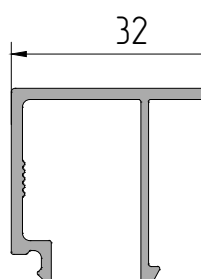
AYPC.C48.0608A Профиль штапика P = 189,1 мм
