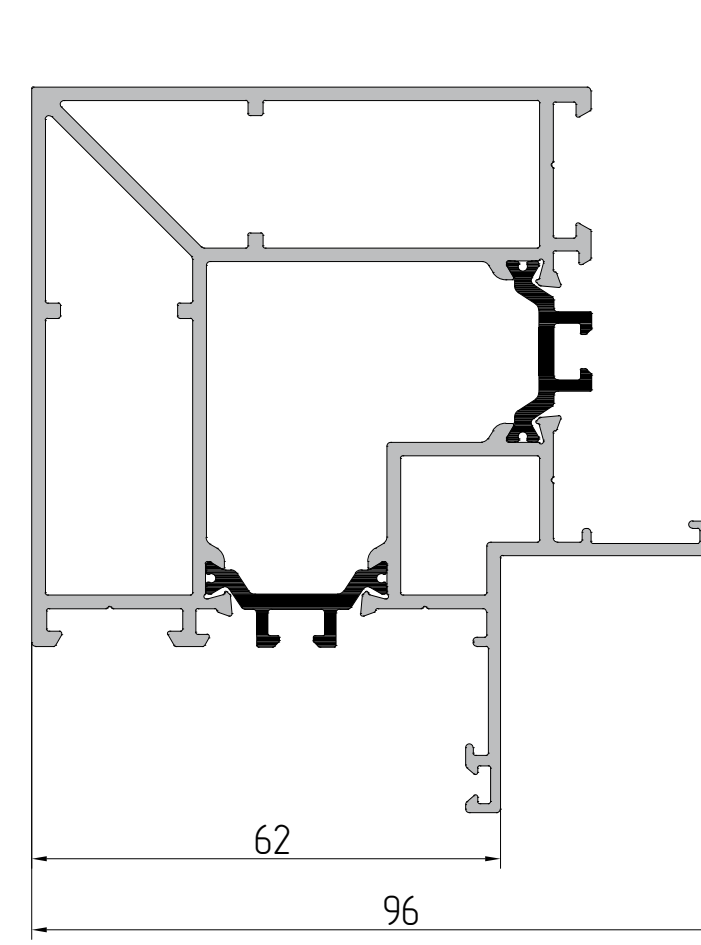
AYPC.W62.0841 Профиль соединителя P = 549 мм J x = 49,0 см² J y = 49,0 см²
