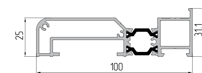
AYPC.W62.0602 Профиль штапика P = 75 мм
