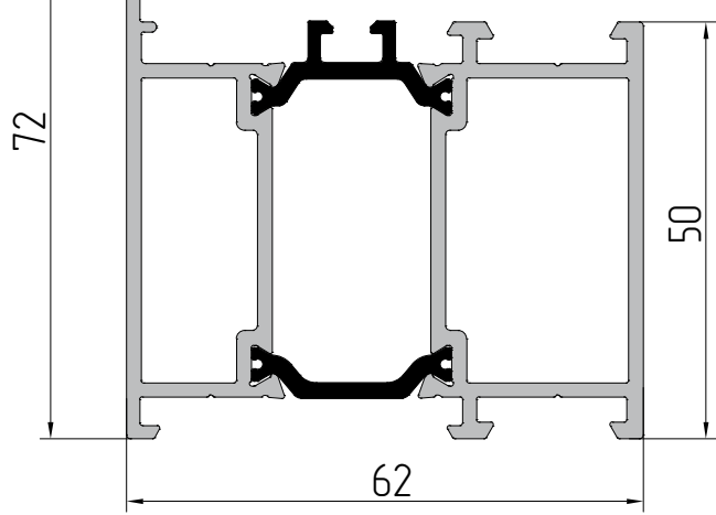
AYPC.W62.0222 Профиль створки P = 436 мм J x = 26,8 см² J y = 14,48 см²
