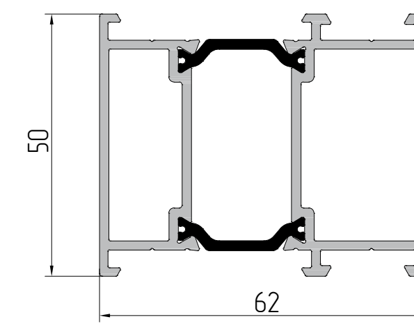
AYPC.W62.0314 Профиль импоста P = 559 мм J x = 41,1 см² J y = 130,8 см²
