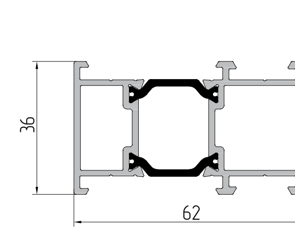
AYPC.W62.0304 Профиль импоста P = 616 мм J x = 148,3 см² J y = 179 см²
