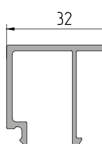
AYPC.C48.0608A Профиль штапика P = 189,1 мм
