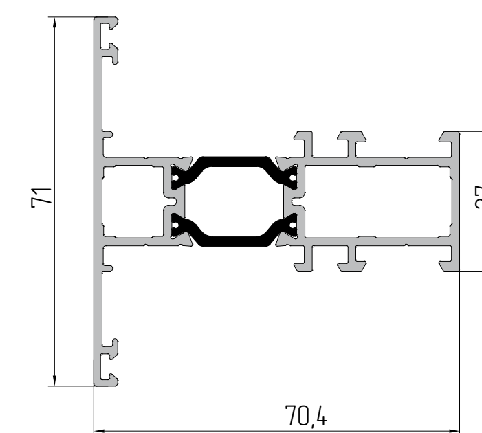
AYPC.W62.0841 Профиль соединителя P = 549 мм J x = 49,0 см² J y = 49,0 см²
