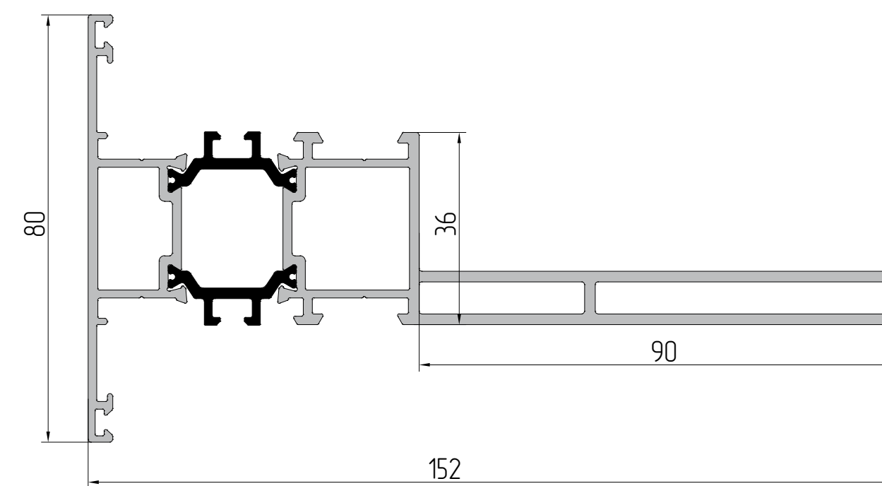
AYPC.W62.0839 Профиль дверной P = 346 мм J x = 21,74 см² J y = 22,21 см²
