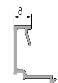
AYPC.C48.0602A Профиль штапика P = 117,7 мм
