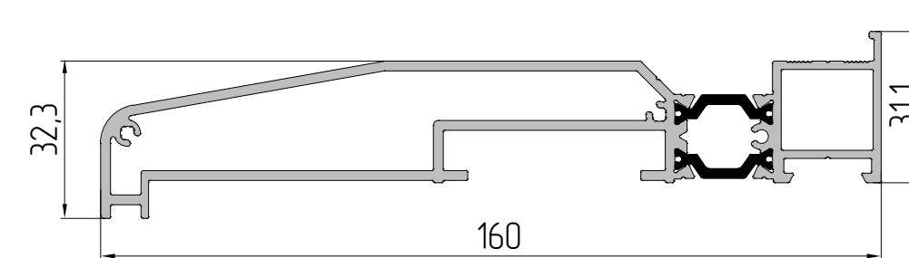
AYPC.W62.0604 Профиль штапика P = 50,8 мм
