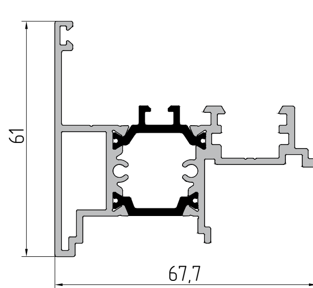
AYPC.W62.0504 Профиль штапика P = 383 мм J x = 15,1 см² J y = 7,5 см²
