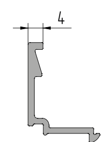
AYPC.C48.0601A Профиль штапика P = 96,1 мм
