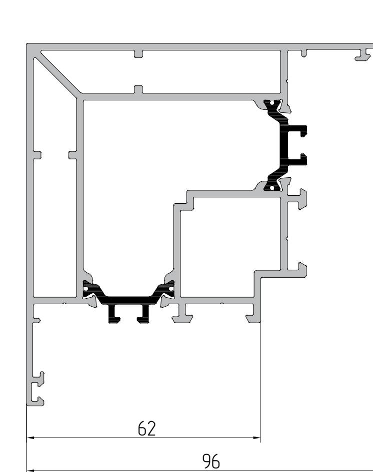
AYPC.W62.0840 Профиль соединителя P = 549 мм J x = 53,0 см² J y = 53,0 см²
