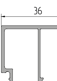
AYPC.C48.0637A Профиль штапика P = 197,3 мм
