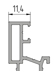
AYPC.W62.0603 Профиль штапика P = 130 мм
