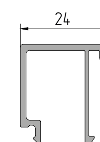
AYPC.C48.0606A Профиль штапика P = 173,1 мм
