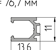
AYPC.F50.0702 Профиль вспомогательный P = 76,7 мм
