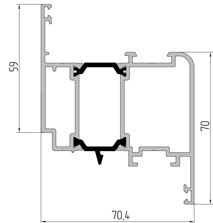
AYPC.W62.0342 Профиль импоста P = 501 мм J x = 41,7 см² J y = 21,5 см²
