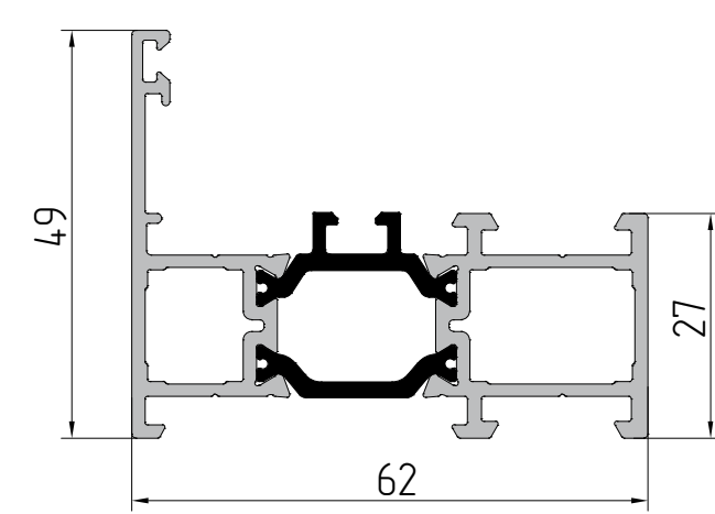
AYPC.W62.0203 Профиль створки P = 441 мм J x = 33,74 см² J y = 28,8 см²
