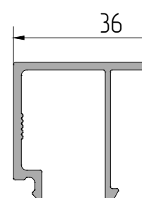
AYPC.C48.0637A Профиль штапика P = 197,3 мм
