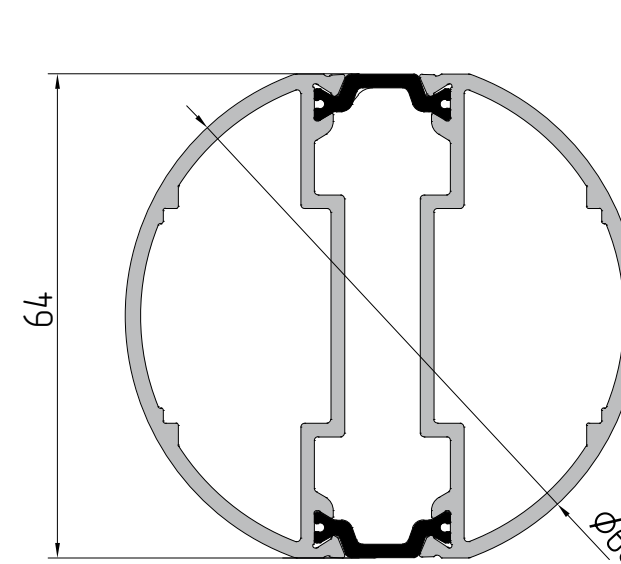
AYPC.W62.0807 Профиль соединителя P = 214 мм J x = 18,9 см² J y = 26,6 см²
