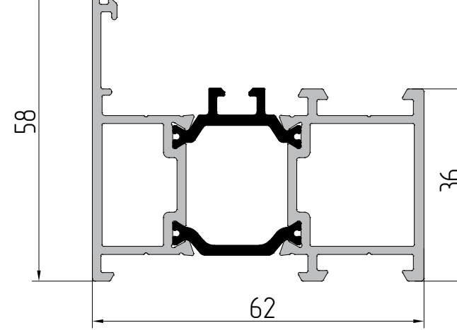
AYPC.W62.0221 Профиль створки P = 418 мм J x = 22,4 см² J y = 8,2 см²
