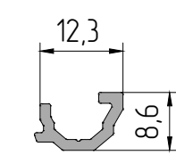
AYPC.W62.0604 Профиль штапика P = 50,8 мм
