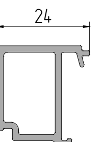
AYPC.C48.2606 Профиль штапика P = 111,5 мм
