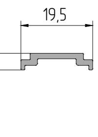
AYPC.W62.0607 Профиль тяги P = 39,2 мм
