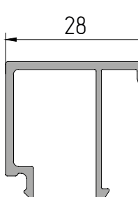
AYPC.C48.0607A Профиль штапика P = 181,1 мм
