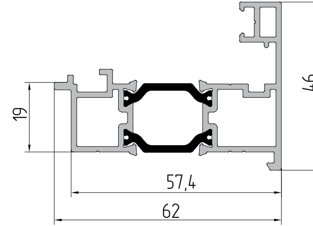
AYPC.W62.0303 Профиль импоста P = 475,7 мм J x = 24 см² J y = 26,3 см²
