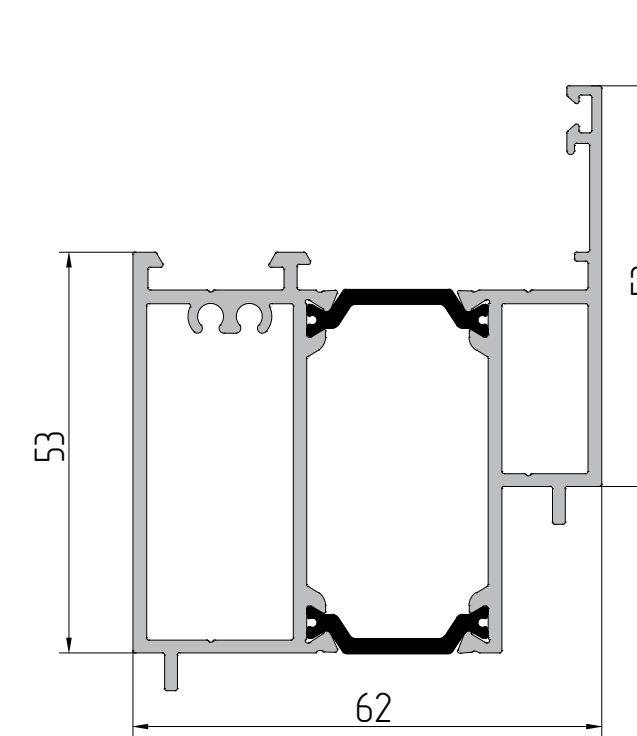
AYPC.W62.0839 Профиль дверной P = 346 мм J x = 21,74 см² J y = 22,21 см²
