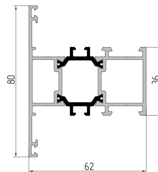
AYPC.W62.0807 Профиль соединителя P = 214 мм J x = 18,9 см² J y = 26,6 см²
