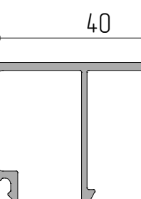
AYPC.C48.0636A Профиль штапика P = 205,3 мм
