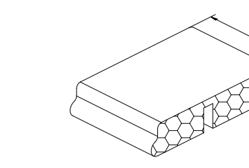
AYPC.W62.0915 (b = 22 мм) AYPC.W62.0915-01 (b = 32 мм) AYPC.W62.0915-02 (b = 45 мм) Подкладка
