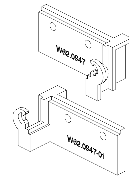
AYPC.W62.0947K Комплект заглушек порога
