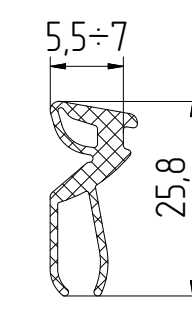
FRK194 Уплотнитель резиновый
