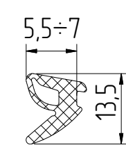
FRK192 Уплотнитель резиновый
