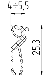
FRK193 Уплотнитель резиновый
