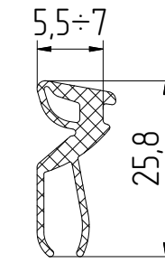
FRK194 Уплотнитель резиновый
