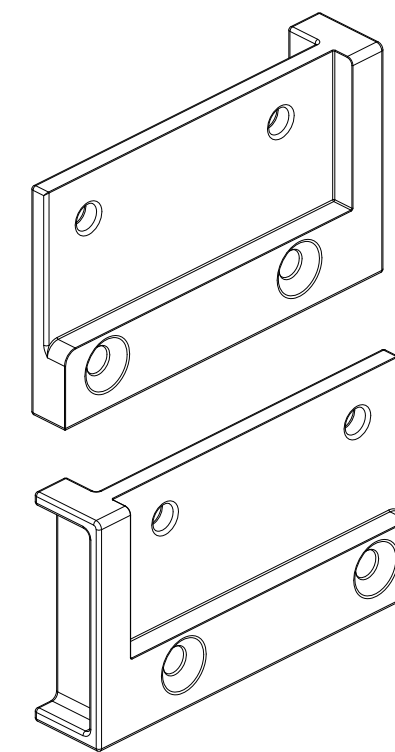
AYPC.W62.9904K Комплект заглушек порога
