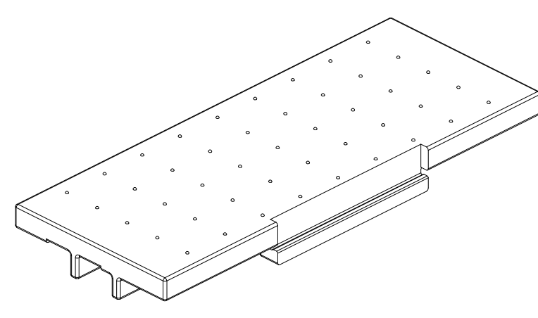
AYPC.C48.0907 Заглушка
