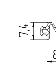
FRK211 Уплотнитель резиновый
