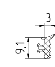
FRK29-01 Уплотнитель резиновый
