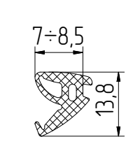
FRK231 Уплотнитель резиновый
