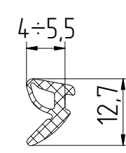
FRK191 Уплотнитель резиновый
