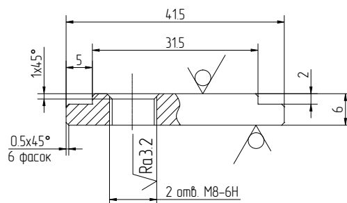
Пластина АУРС.С48.0944
