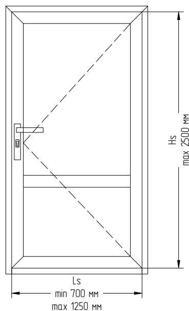
открывание внутрь
