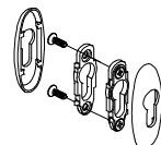
Накладка на цилиндр арт.1031.04 (Stublina)
