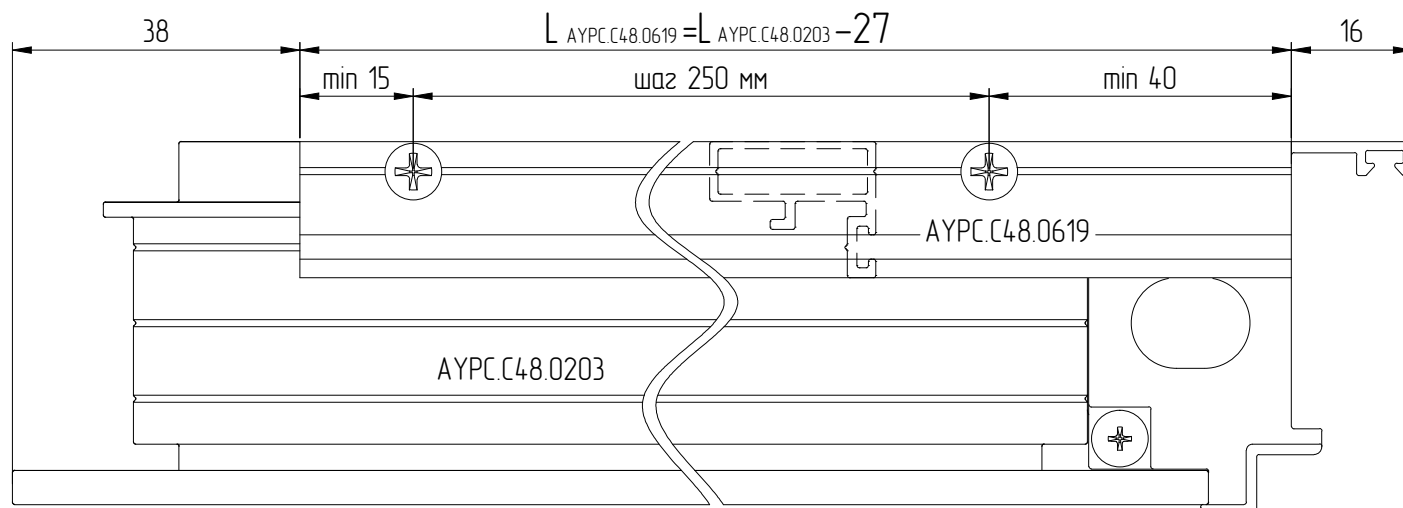
Схема установки профиля АУРС.С48.0619
