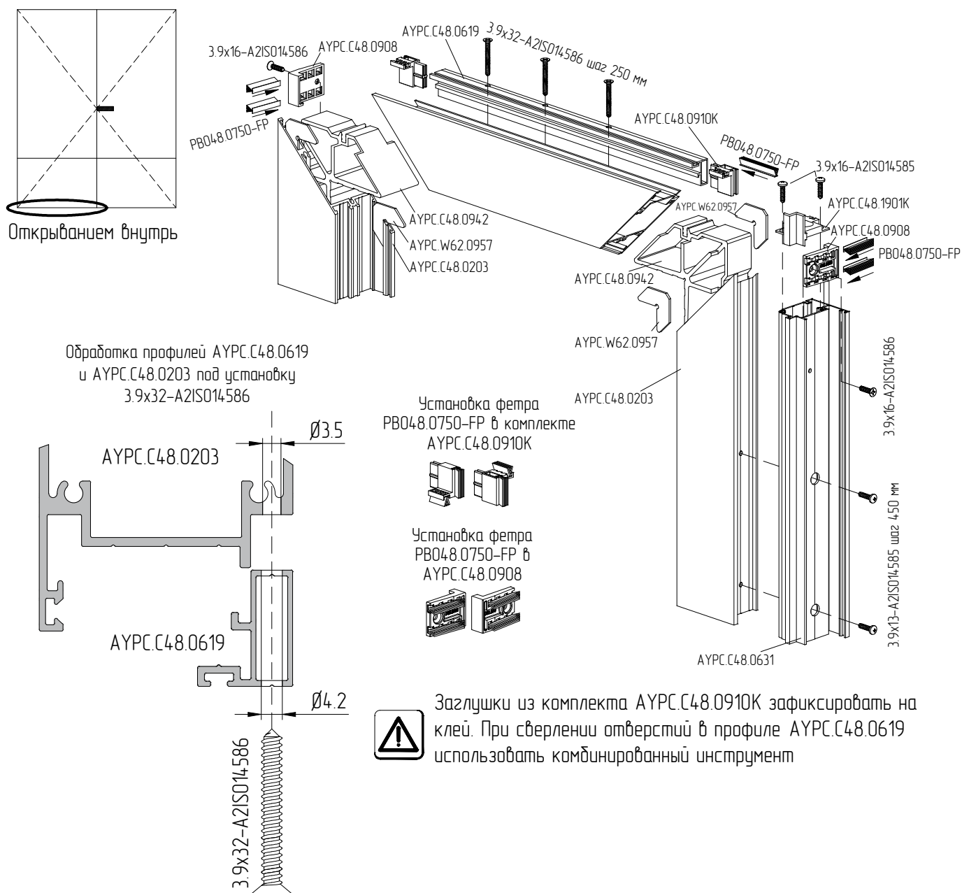
Схема установки профиля АУРС.С48.0619
