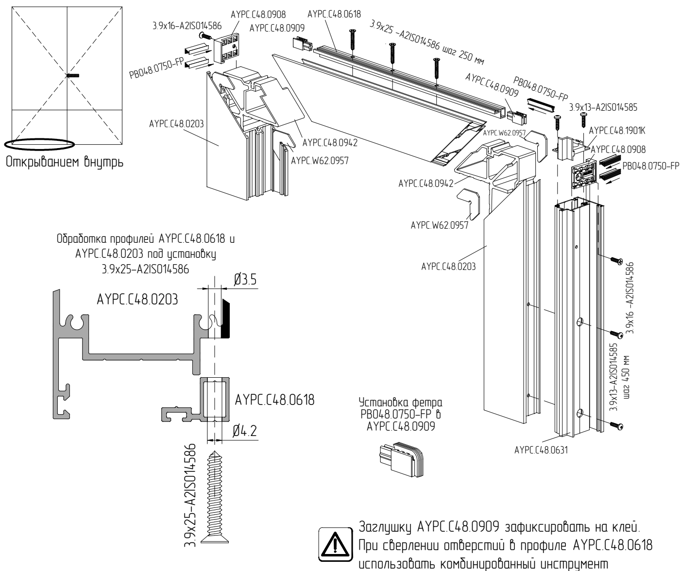
Схема установки профиля АУРС.С48.0618
