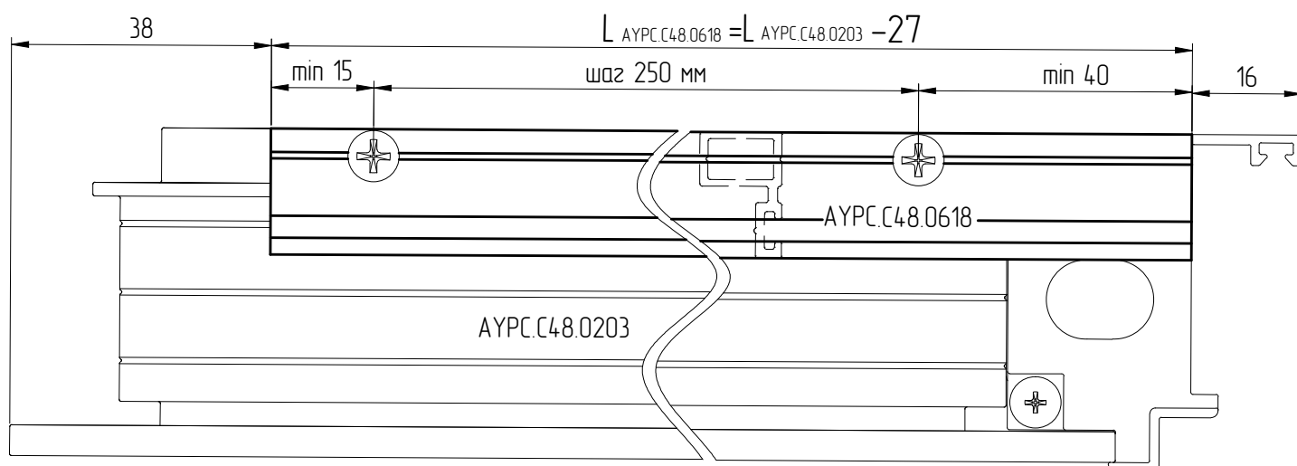
Схема установки профиля АУРС.С48.0618
