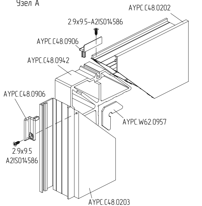
Узел А
