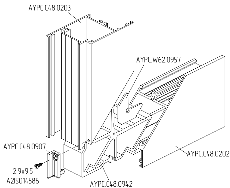
Узел Б
