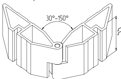
Закладная угловая АУРС.У62.0962-04
