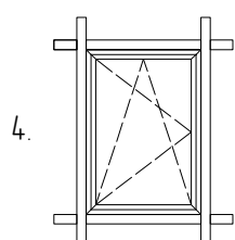
Поворотно-откидное окно в фасад F50/F60
