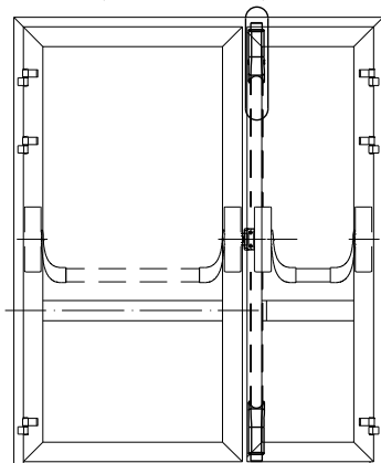
Трехточечное запирание
