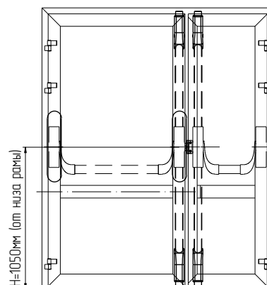
Пятиточечное запирание
