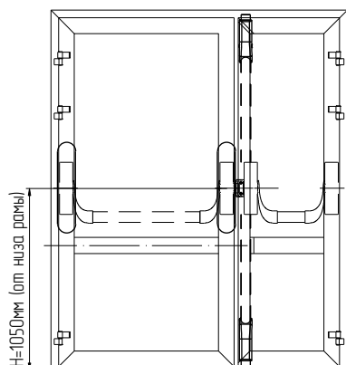
Трехточечное запирание
