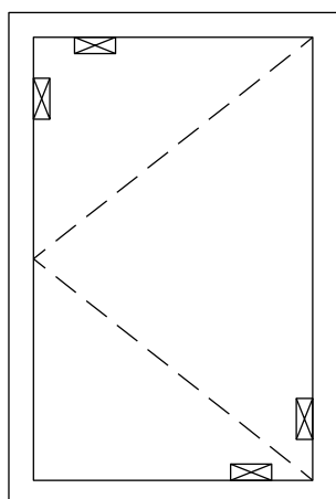
Поворотное окно
