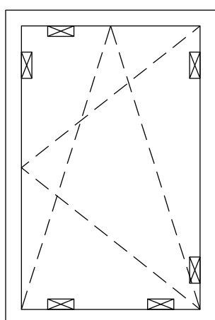
Поворотно-откидное окно
