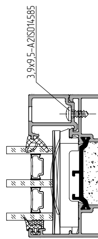
Схема крепления профиля штапика винтами самонарезающими 3,9x9,5-A2IS014585
