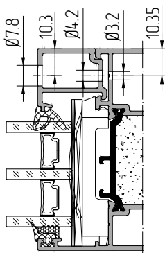
Схема обработки профилей под установку винта самонарезающего 3,9x9,5-A2IS014585
