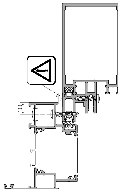
Схема крепления профиля спецами
