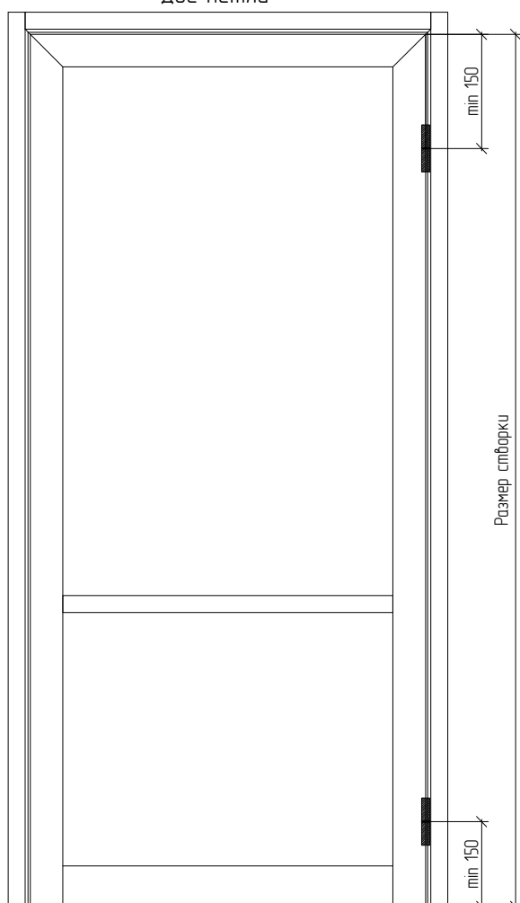
Рекомендуемые схемы установки петель
