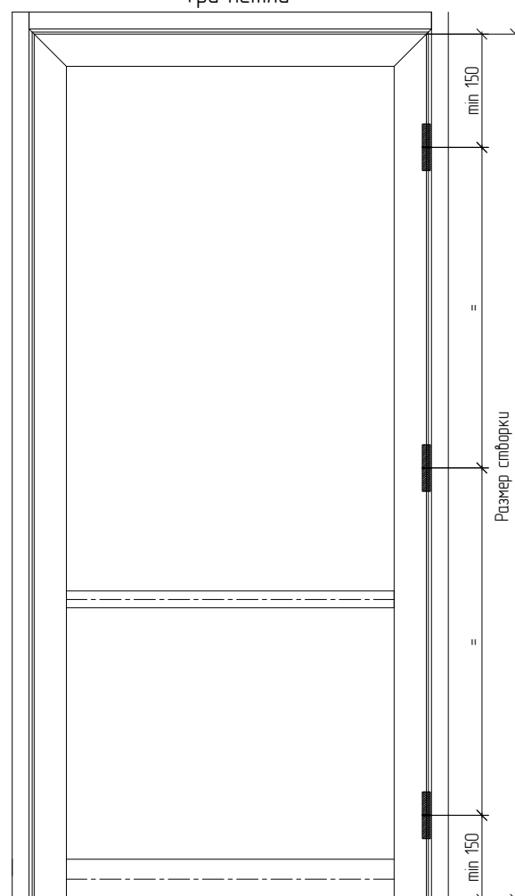
Рекомендуемые схемы установки петель
