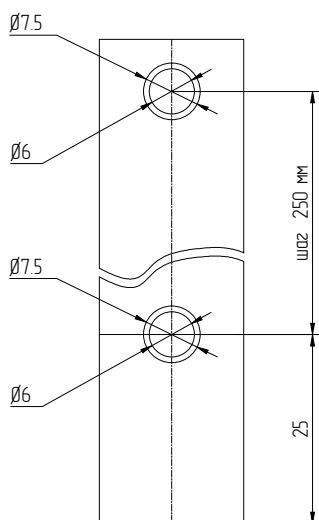
Обработка профиля АУРС.118.0001 под ВС 3,9х16-А2IS014586
