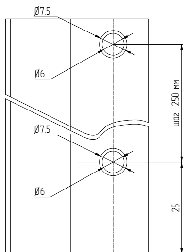
Обработка профиля АУРС.118.0004 под ВС 3,9х16-А2IS014586
