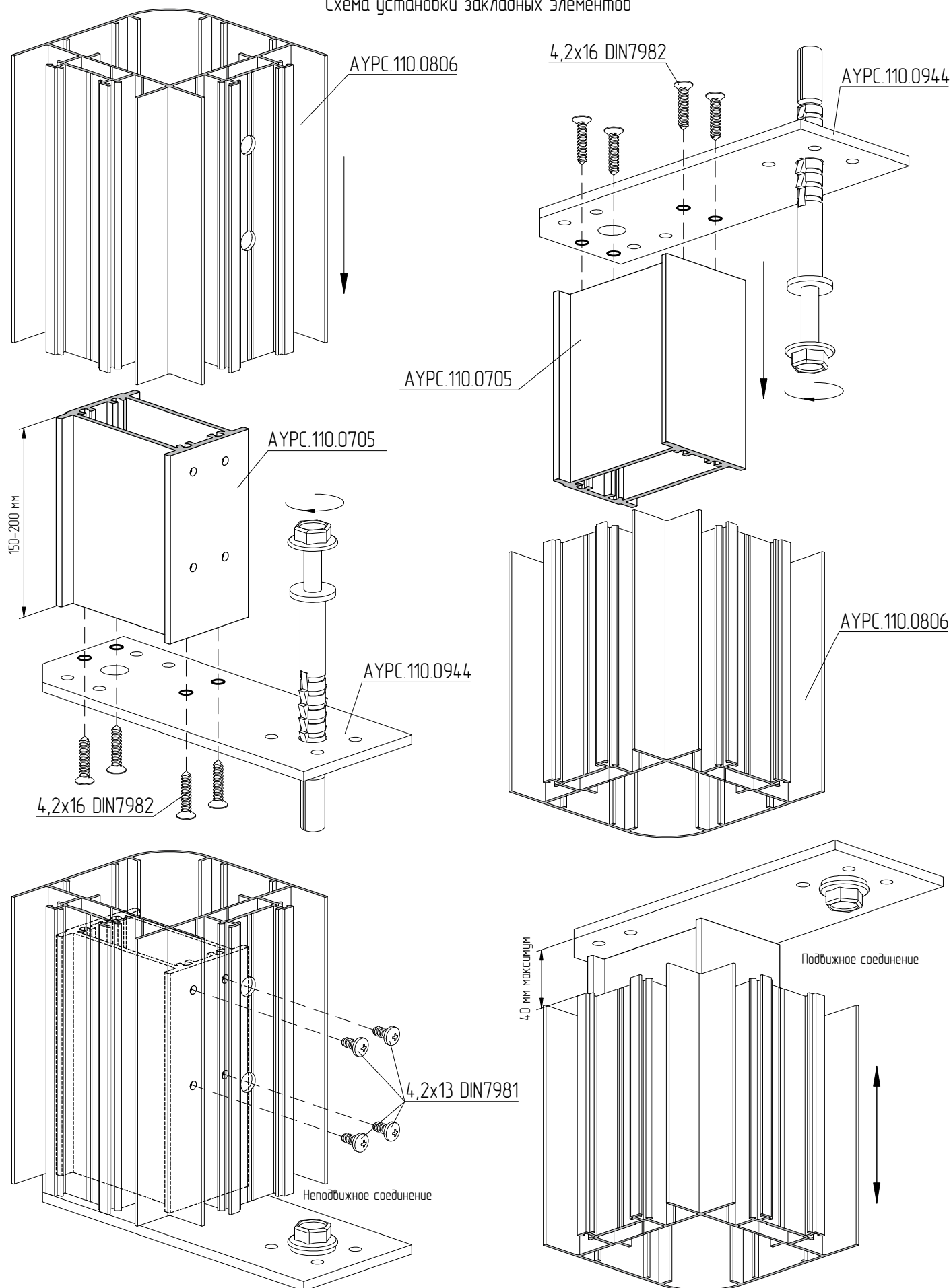
Схема установки закладных элементов
