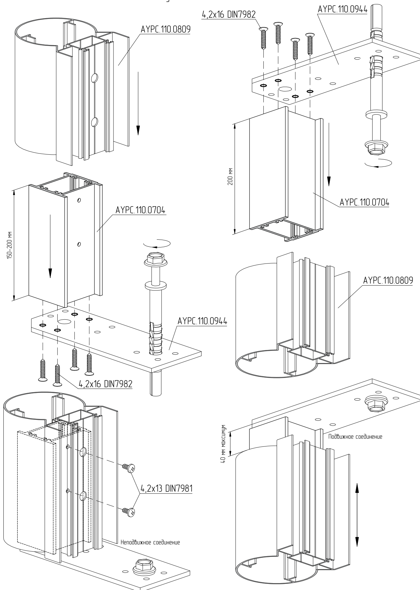
Схема установки закладных элементов
