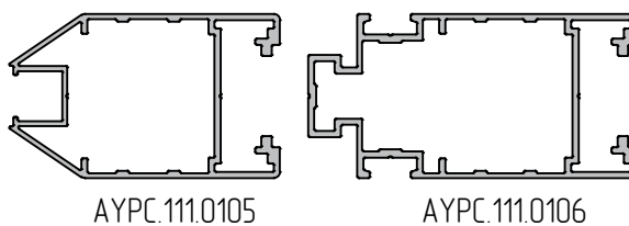
вариант для установки уголка MONO406
