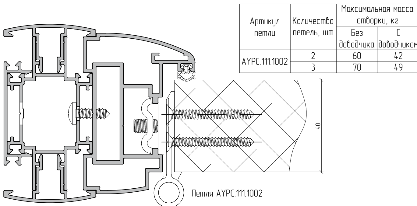
Схема установки петель на деревянную створку двери
