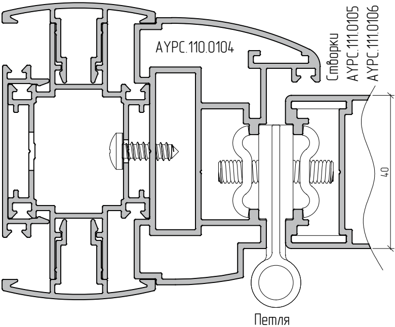
Рекомендуемые схемы установки петель
