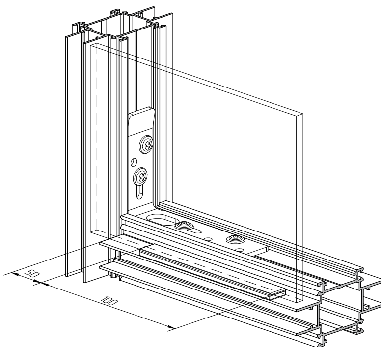
Распашная дверь
