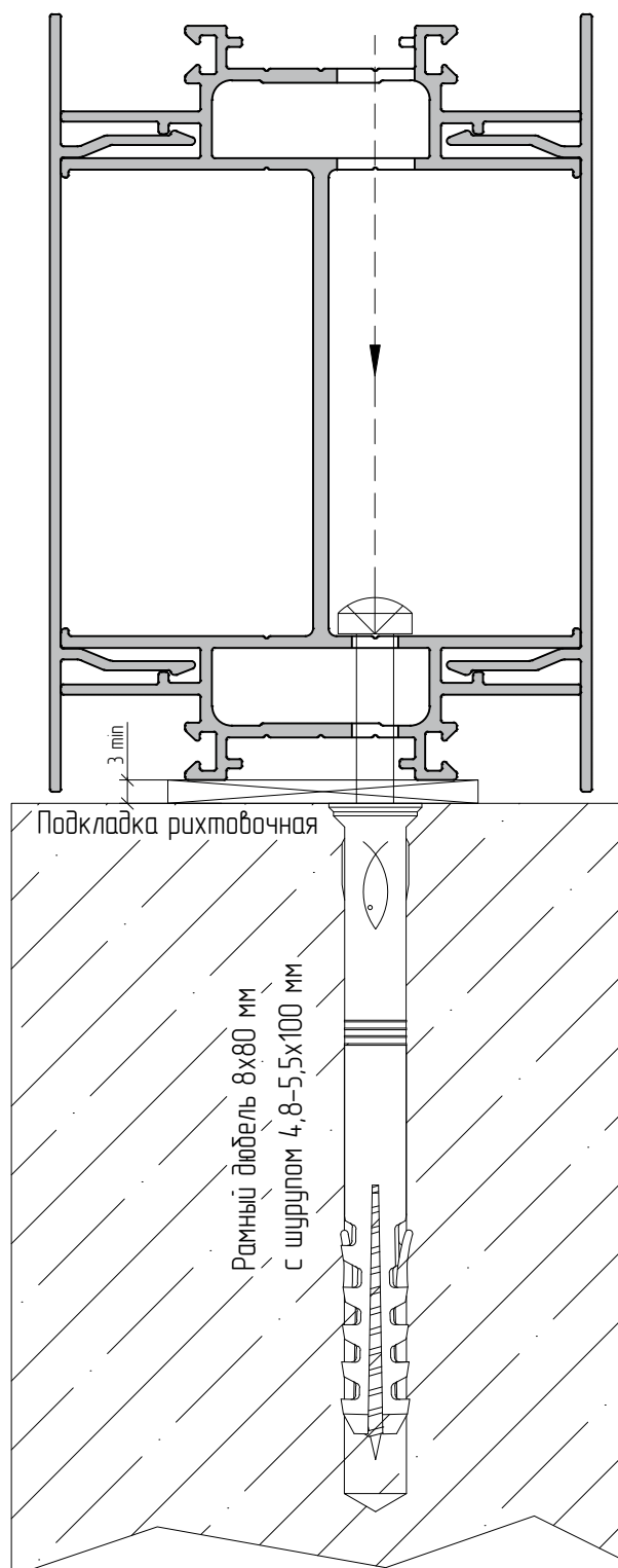
Крепление профиля AYPC.110.0304 к перекрытию
