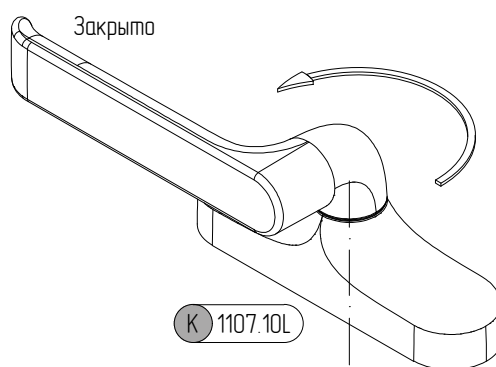
2.4.2. Положение левой оконной ручек Stublina-состояние Открыто/Закрыто
