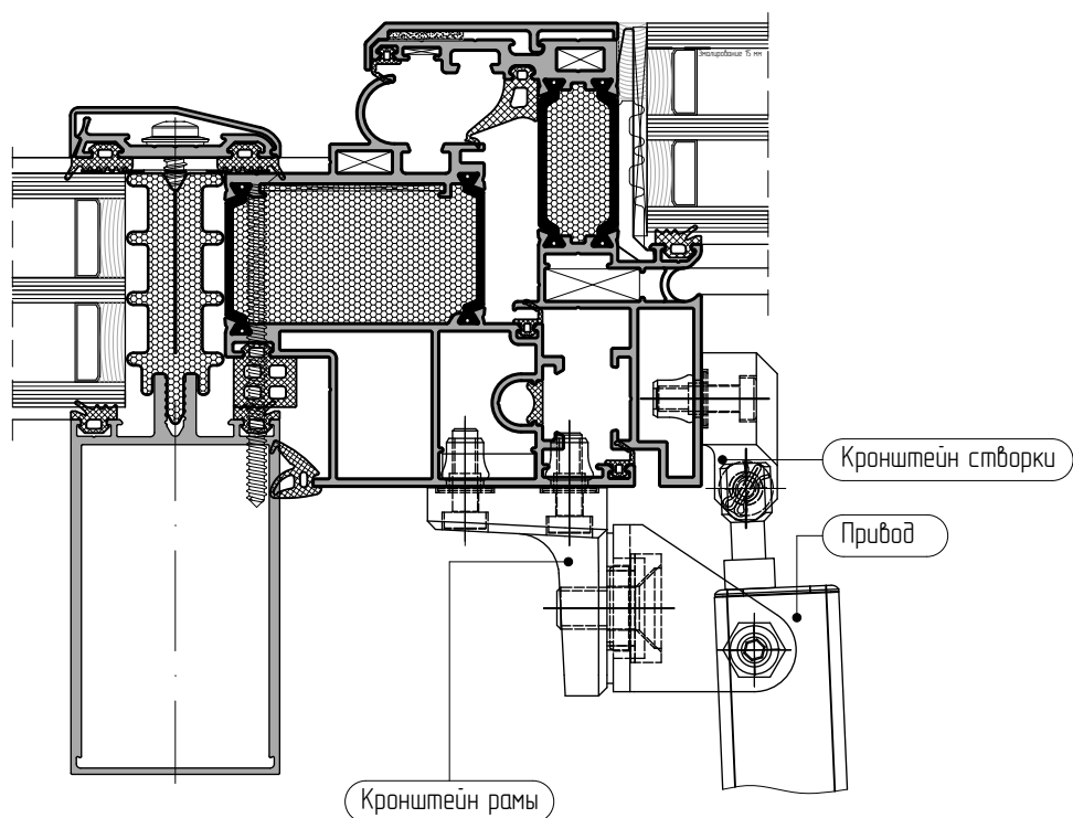
Пример установки электрического привода с кронштейнами
