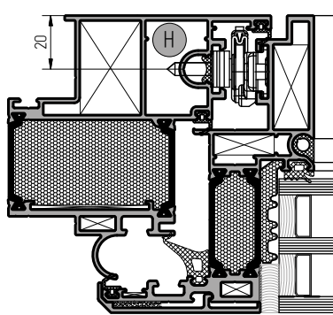
Установка ограничителя открывания арт. 4065.00
