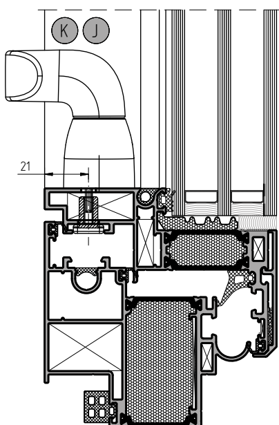
Установка поводковой ручки арт.1107.10R и арт.1107.10L
