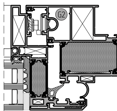
Установка ответной планки арт. 4010.80
