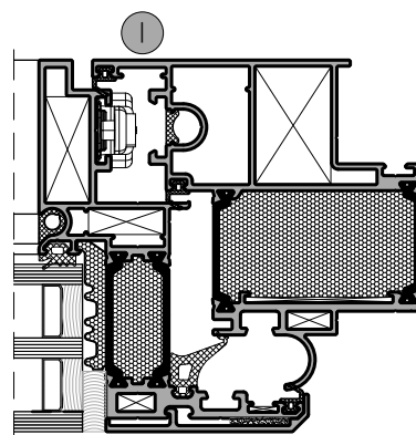
Установка углового переключателя арт. 4010.20
