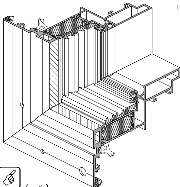
Створка Тип №3
