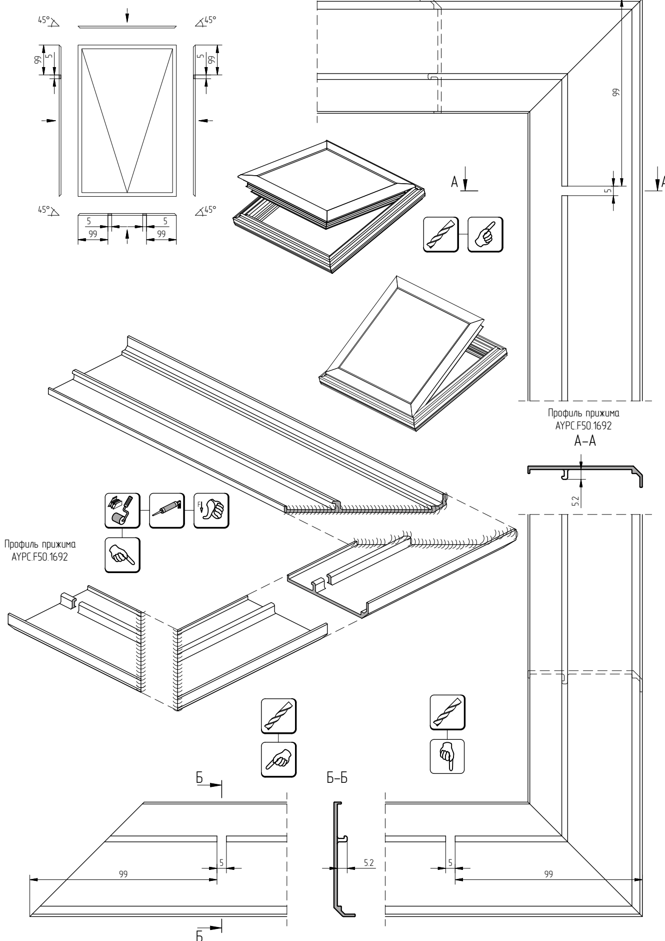
Створка Тун №1
