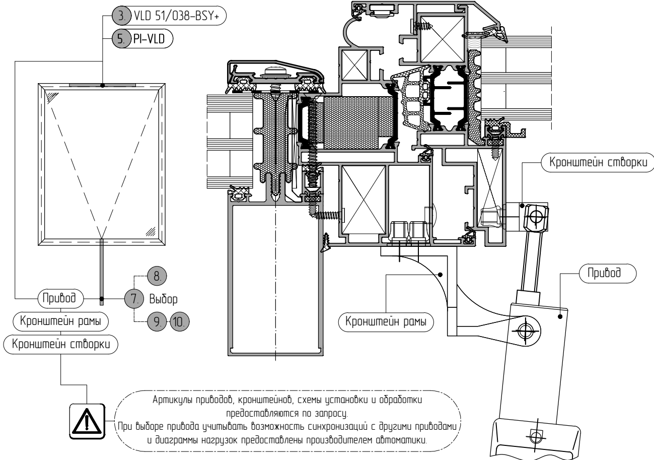
Примеры установки электрических приводов с кронштейном
