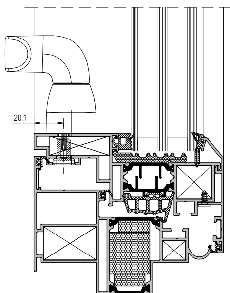
Установка поводковой ручки арт.1107.10R и арт.1107.10L
