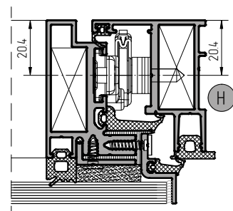
Установка ограничителя открывания арт. 4065.00
