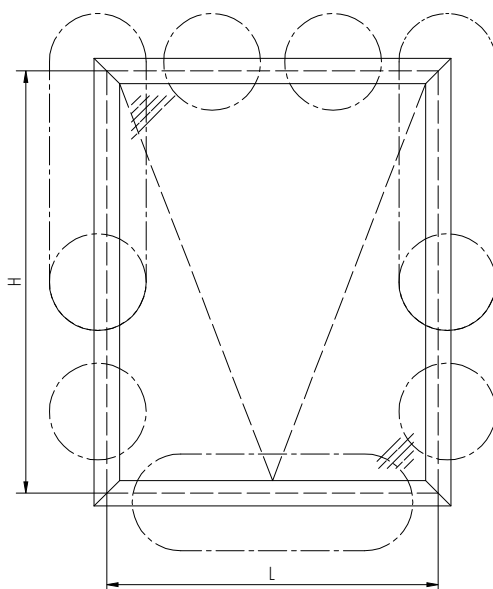
Установка поводковой ручки арт.1107.10R и арт.1107.10L
