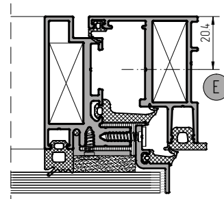
Установка механизма регулировки по высоте арт.4060.04
