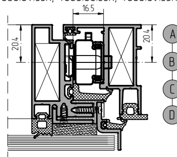
Установка фрикционных ножиц арт. 4060.07.55R, 4060.08.55R, 4060.09.55R
