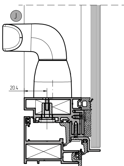
Установка поводковой ручки арт.1107.10R и арт.1107.10L
