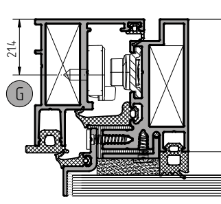
Установка ответной планки арт. 4060.10.50
