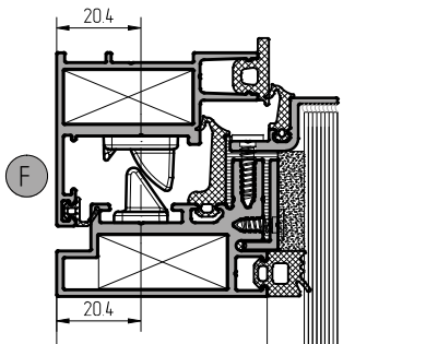
Установка скрытого верхнего прижима арт. 4060.45
