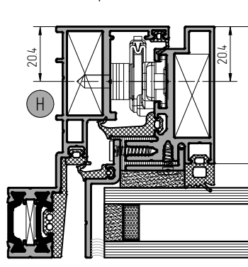
Установка ограничителя открывания арт. 4065.00
