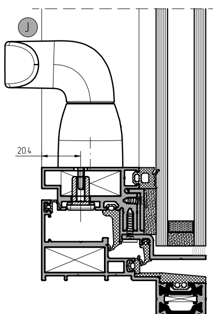
Установка поводковой ручки арт.1107.10R и арт.1107.10L
