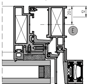
Установка механизма регулировки по высоте арт.4060.04
