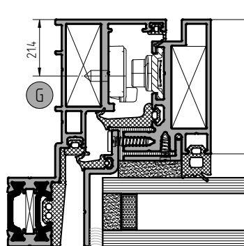
Установка ограничителя открывания арт. 4065.00
