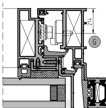
Установка ограничителя открывания арт. 4065.00
