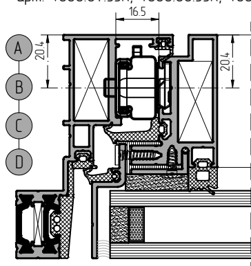
Установка фрикционных нажниц арт. 4060.07.55R, 4060.08.55R, 4060.09.55R
