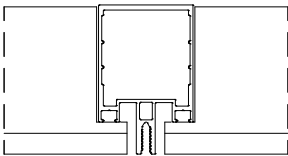
Ригель внахлест
