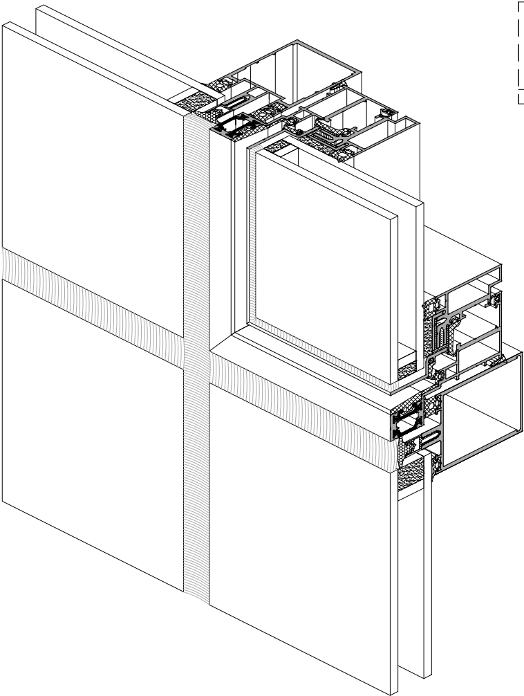
Ригель внахлест
