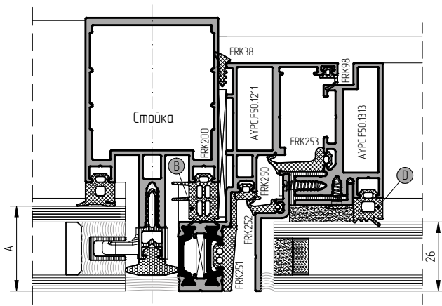
Сечение через стойку
