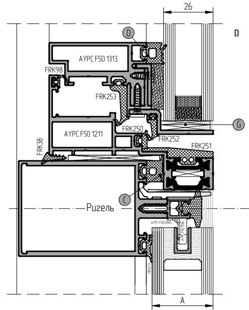
Сечение через ригель
