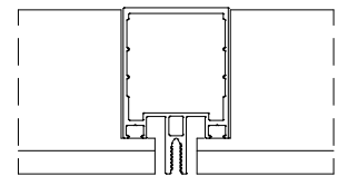
Ригель внахлест
