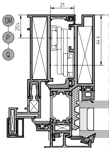
Установка поводковой ручки арт. 1107.10L
