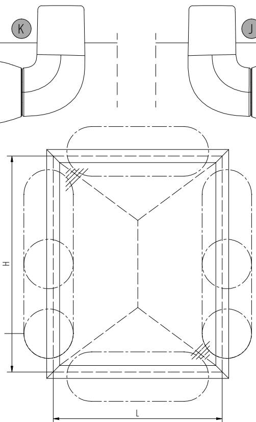
Установка параллельно-отставных ножиц арт. НС820-19L, НС820-28
