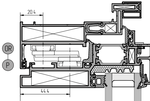
Установка параллельно-отставных ножиц арт. НС820-19R, НС820-28
