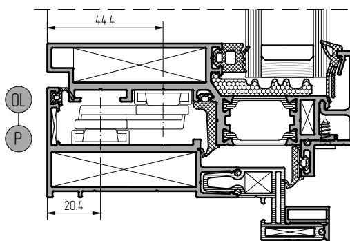
Установка параллельно-отставных ножиц арт. НС820-19L, НС820-28
