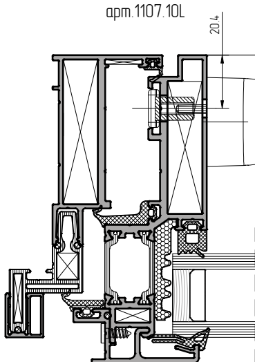
Установка поводковой ручки арт. 1107.10L
