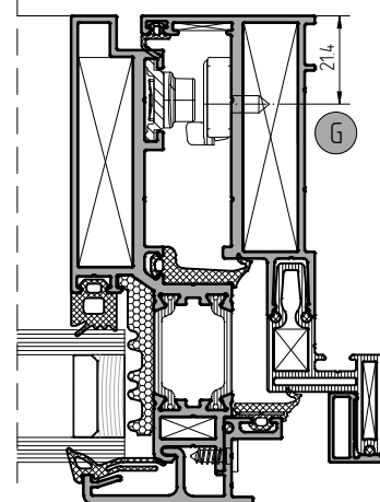
Установка ответной планки арт. 4060.10.50
