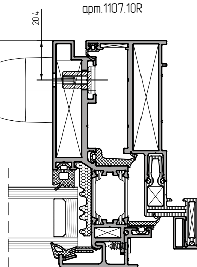
Установка поводковой ручки арт. 1107.10R
